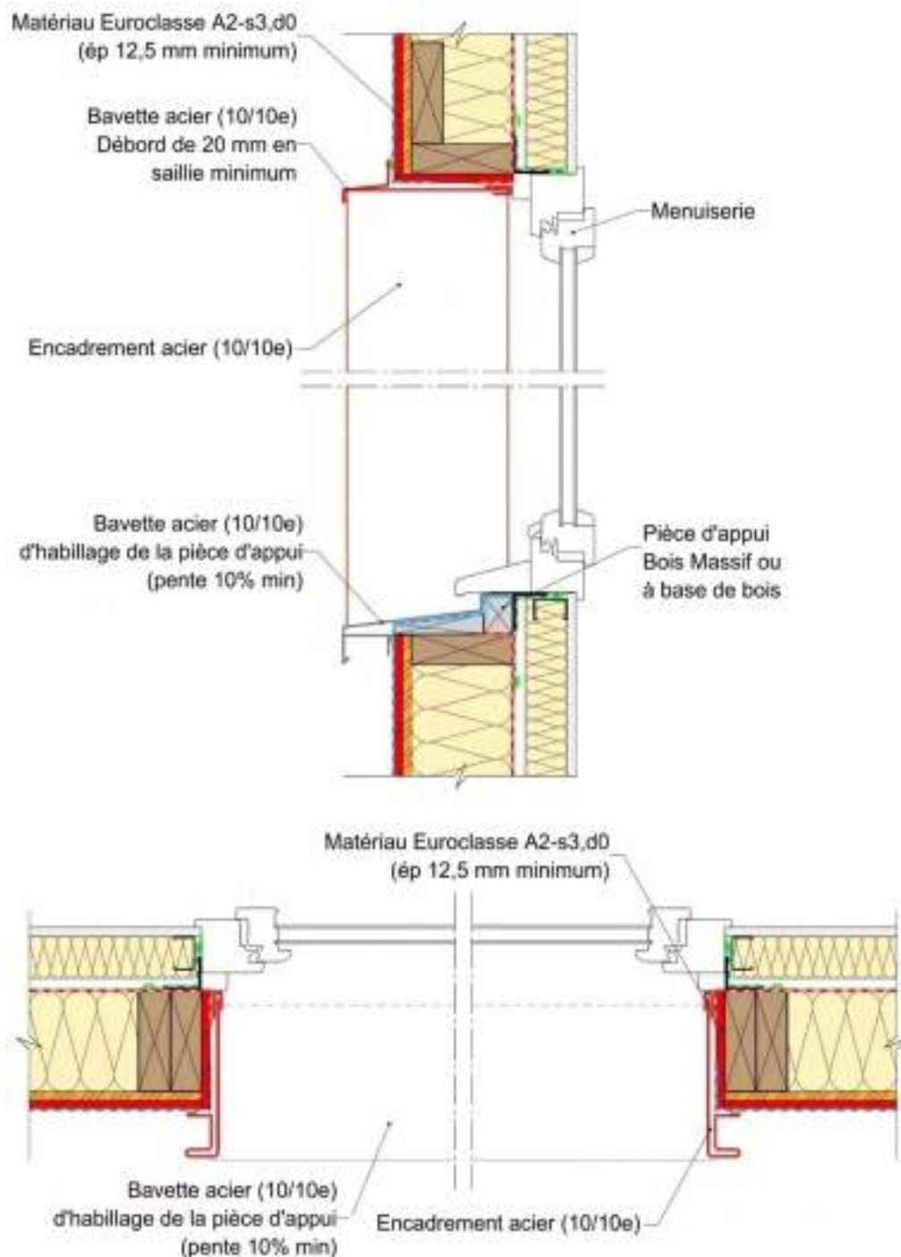
Figure A1.2 : Coupe verticale et horizontale de l'encadrement des baies
