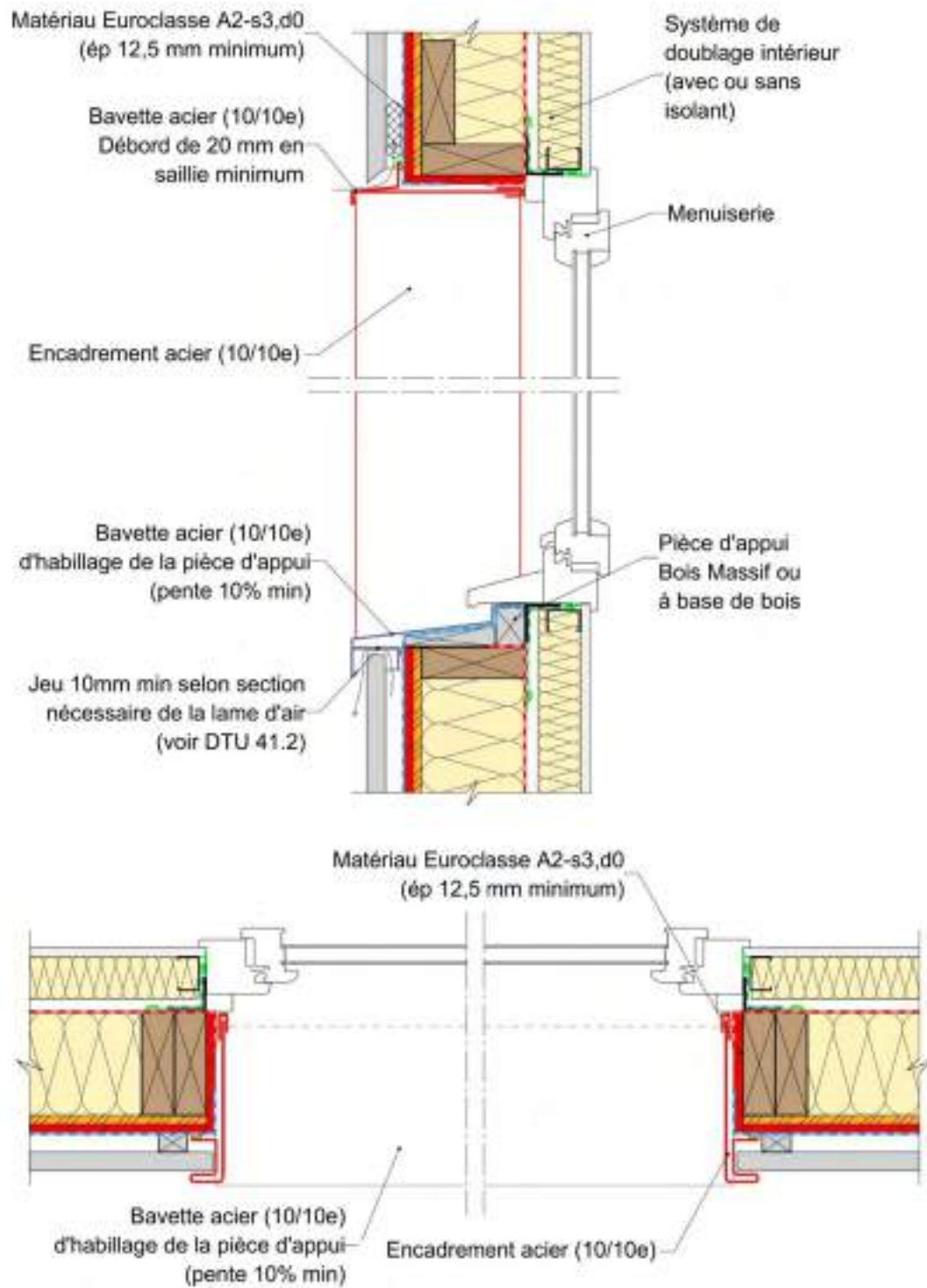
Figure 6: Traitement des baies - menuiseries en applique intérieure avec un matériau A2-s3, d0 + encadrement acier.
