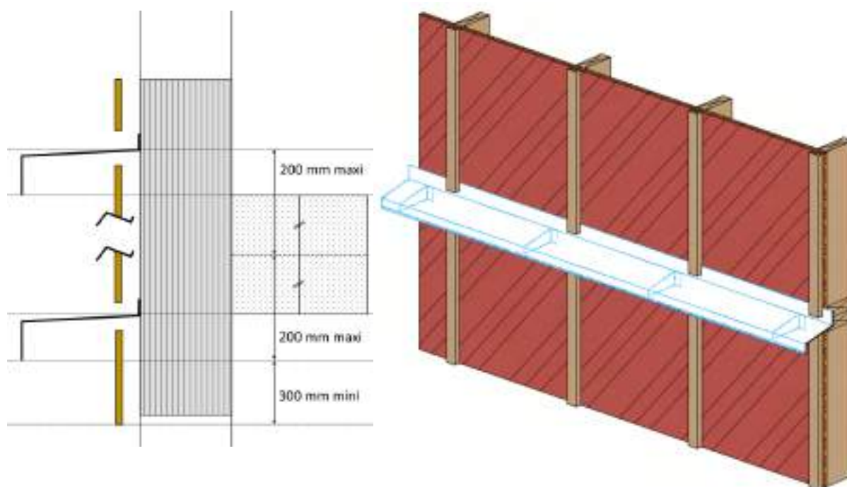
Figure 15: Géométrie, positionnement et mise en œuvre des déflecteurs de flamme.
