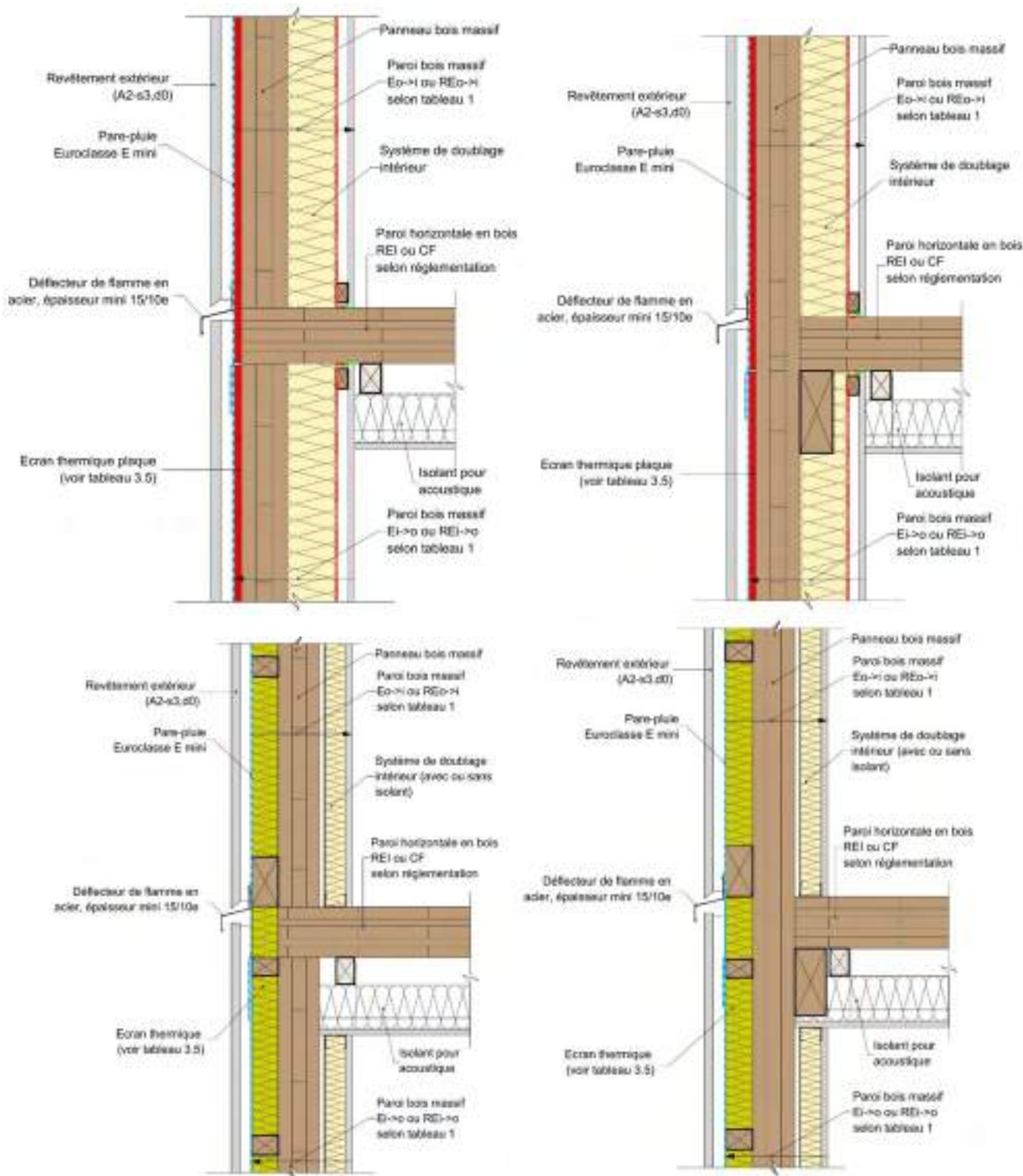
Figure 40 : Façade/mur en panneaux bois massif et plancher en panneaux bois massif.
