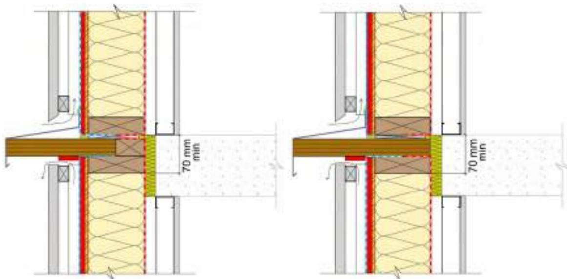
Figure 18 : Principe de configuration du déflecteur renforcé
