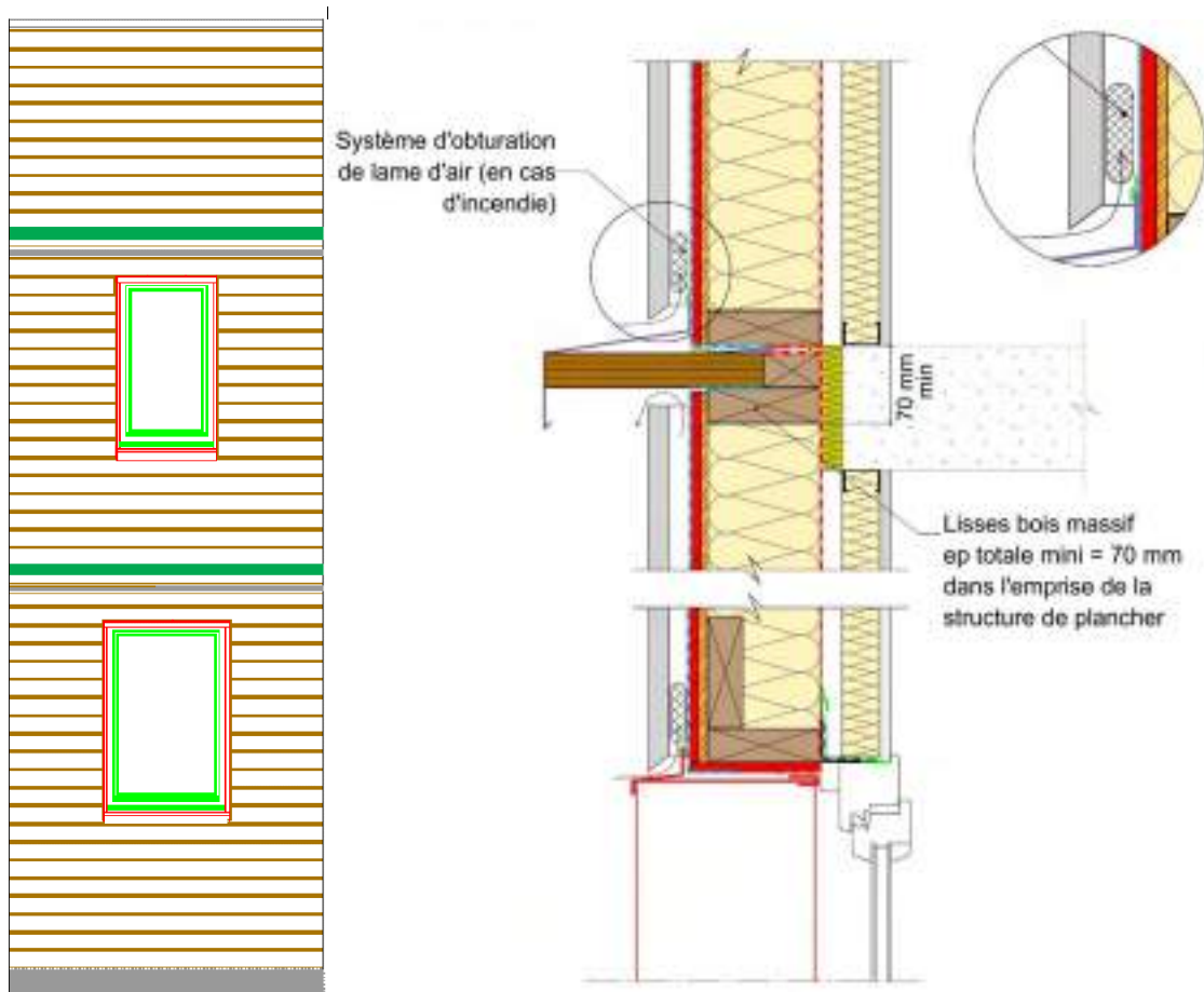
Figure 14 : Position des dispositifs d'obturation de la lame d'air si la durée de résistance au feu de la structure est inférieure ou égale à 60 minutes avec un bardage ventilé dont la performance en réaction au feu du parement est soit de classe D-s2, d0 ou soit de classe C-s2, d0
