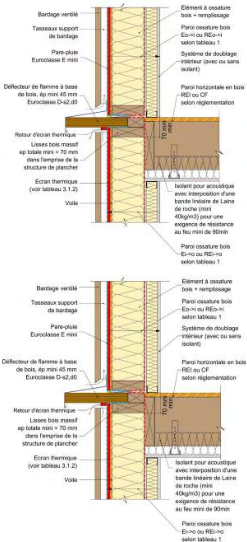
Figure 27 : Exemple de paroi avec déflecteurs renforcés d'une façade/mur ossature bois et plancher en ossature bois.
