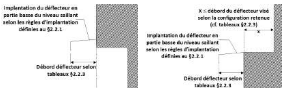
Figure 20 : Décalage du niveau supérieur vers l'extérieur (encorbellement) et vers l'intérieur (retrait) lorsque la distance X est inférieure ou égale au débord du déflecteur du tableau du §2.2.3
