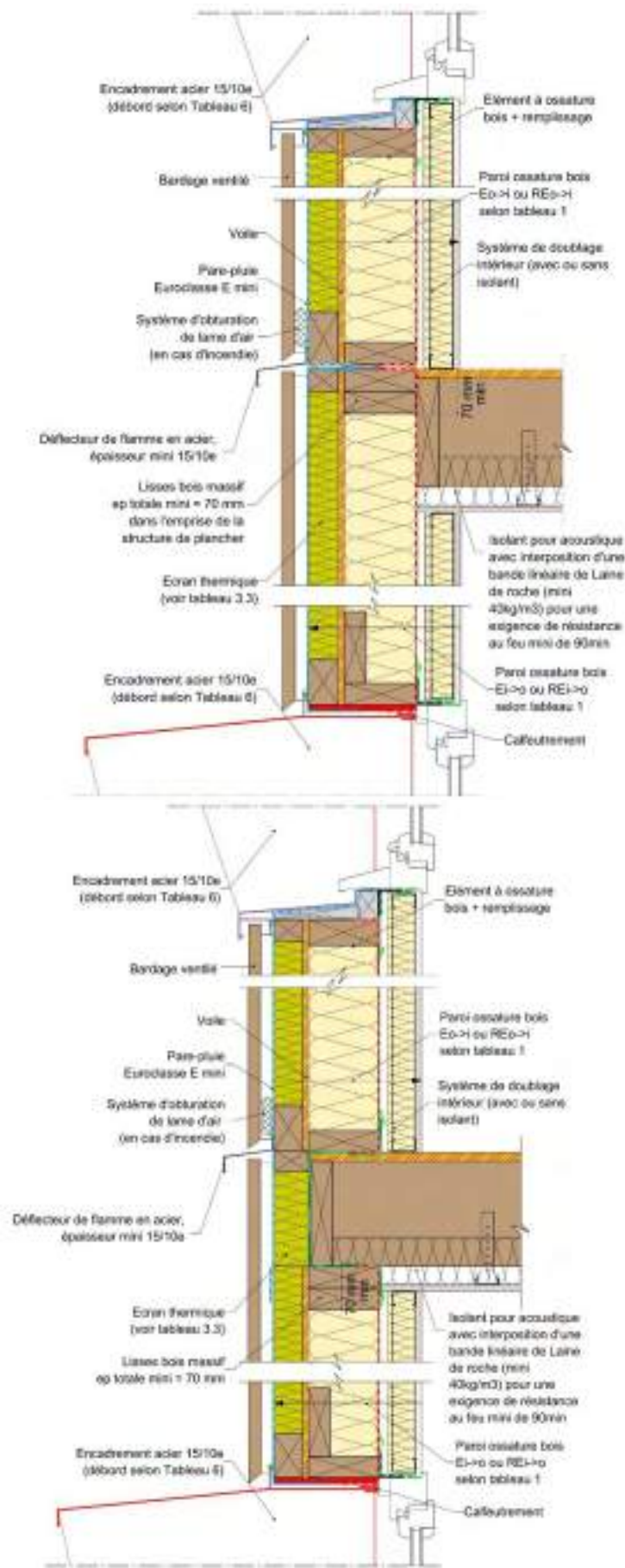
Figure 35 : Façade/mur en ossature bois et plancher en ossature bois.
