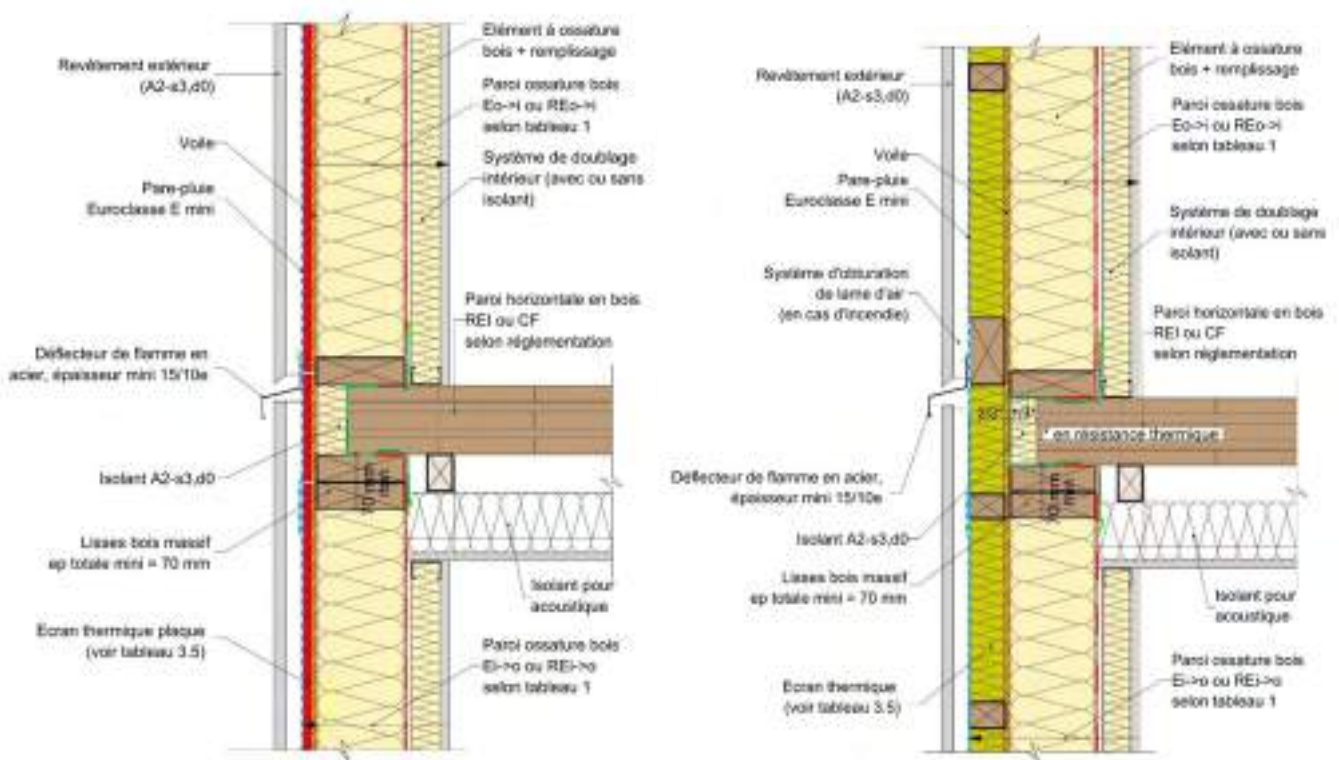
Figure 41 : Façade/mur en ossature bois et plancher en panneaux bois massif.
