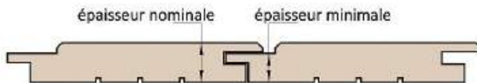
Figure 13: Définition des épaisseurs sur un exemple de profil de bardage.
