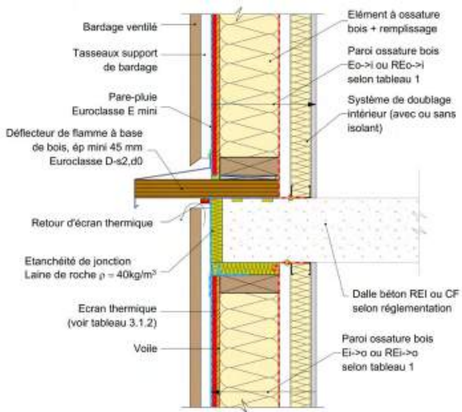
Figure 28 : Exemple de paroi avec déflecteurs renforcés d'une façade ossature bois et plancher en béton.
