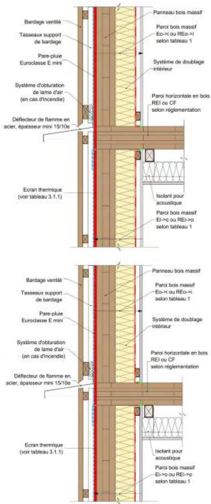
Figure 24 : Façade/mur en panneaux bois massif contrecollés et contrecloués et plancher en panneau bois massif contrecollés et contrecloués.
