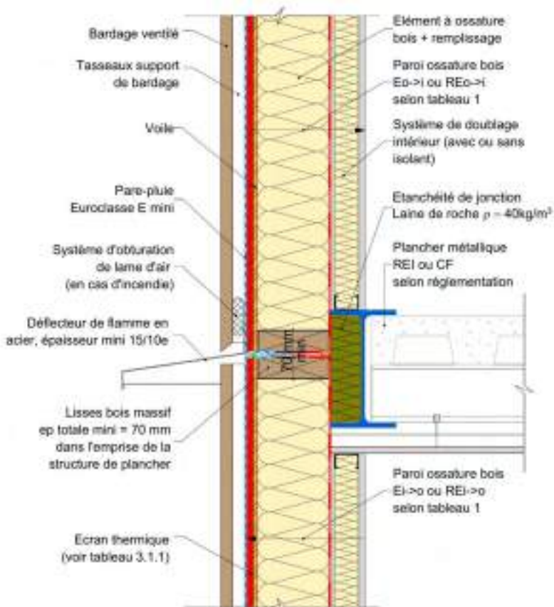
Figure 26 : Façade/mur ossature bois et plancher métallique.
