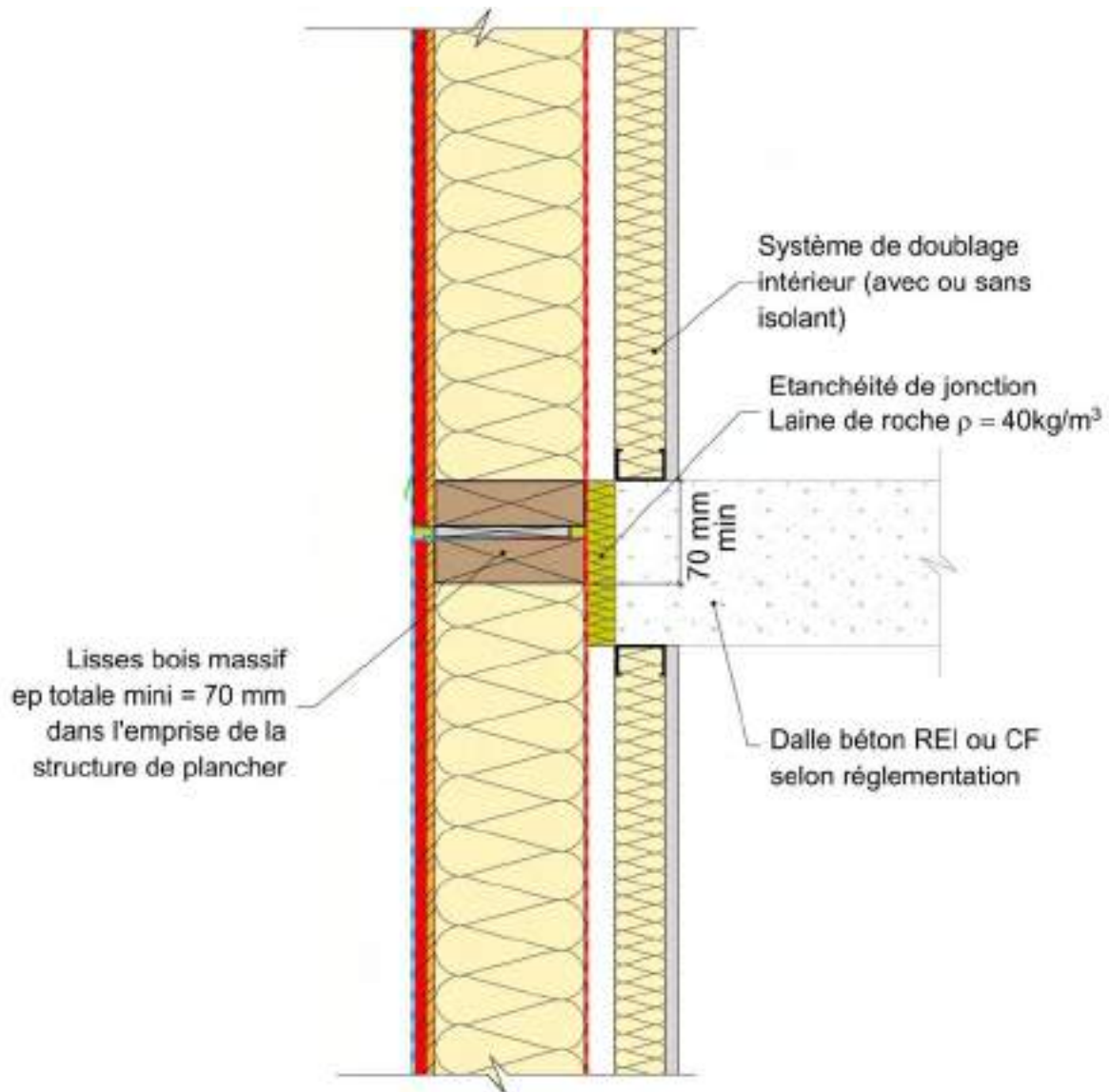
Figure A1.3 : Jonction Façade - plancher
