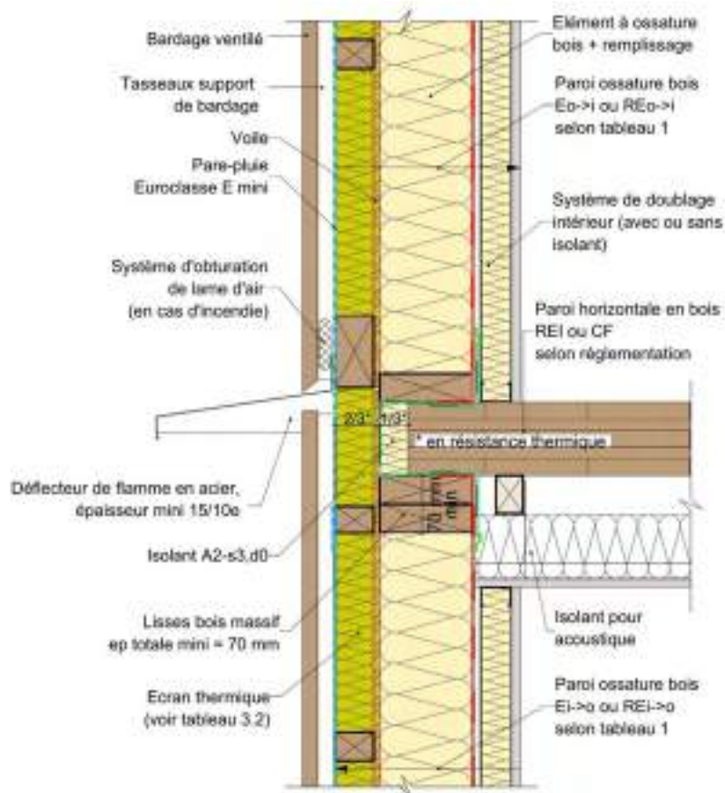
Figure 32 : Façade/mur ossature bois et plancher en panneau bois massif.
