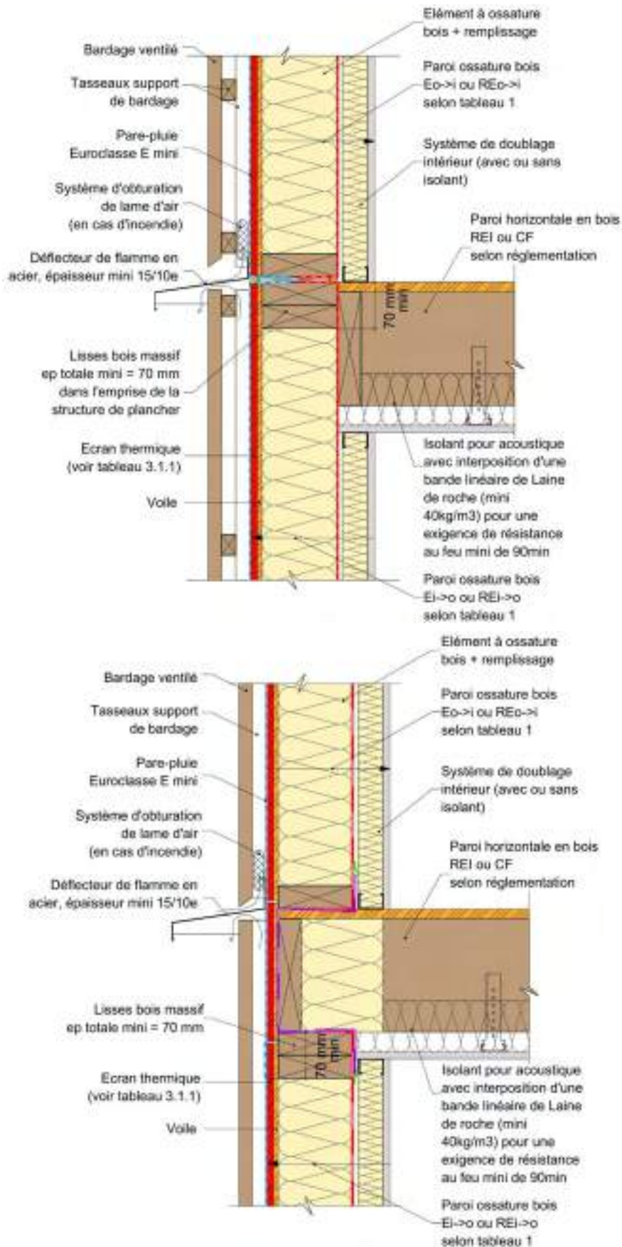
Figure 23 : Façade/mur ossature bois et plancher en ossature bois.
