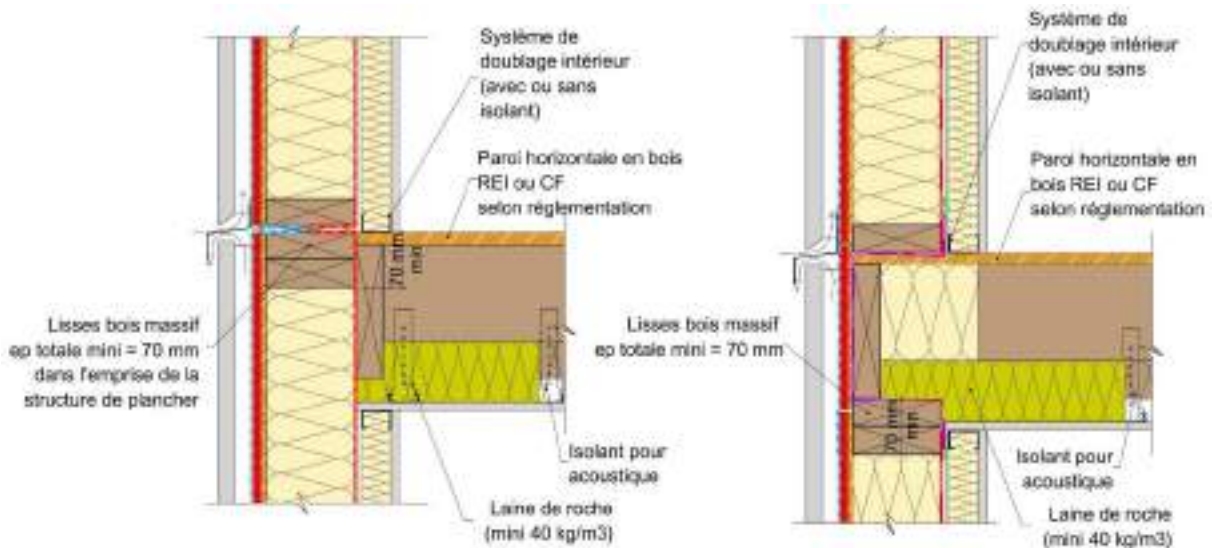
Figure 4: Traitement de l'étanchéité au nez d'un plancher bois avec doublage intérieur assurant l'intégralité de l'exigence EI_{i \rightarrow o} requise et au moins égale à la performance du plafond (si la durée de résistance au feu de la structure est supérieure ou égale à 90 minutes).
