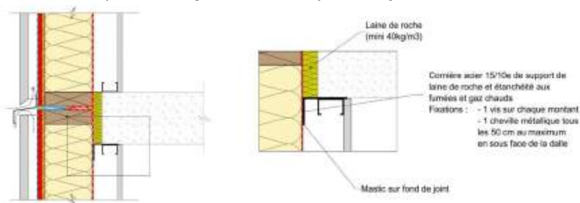
Figure 2: Traitement de l'étanchéité au nez de dalle béton (si la durée de résistance au feu de la structure est supérieure ou égale à 90 minutes).
