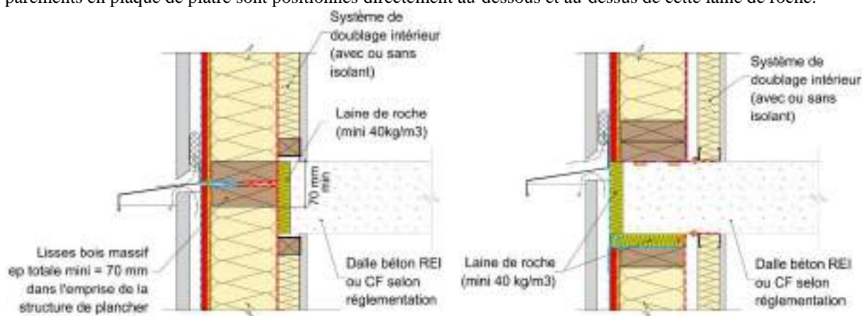
Figure 1: Traitement de l'étanchéité au nez de dalle béton (si la durée de résistance au feu de la structure est inférieure ou égale à 60 minutes).
