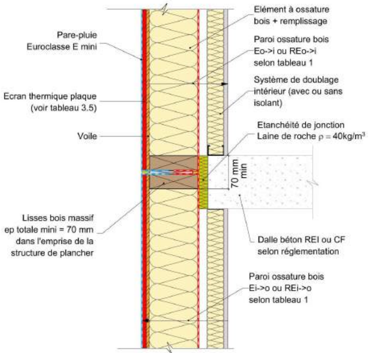
Figure A1.1 : paroi type, partie courante
