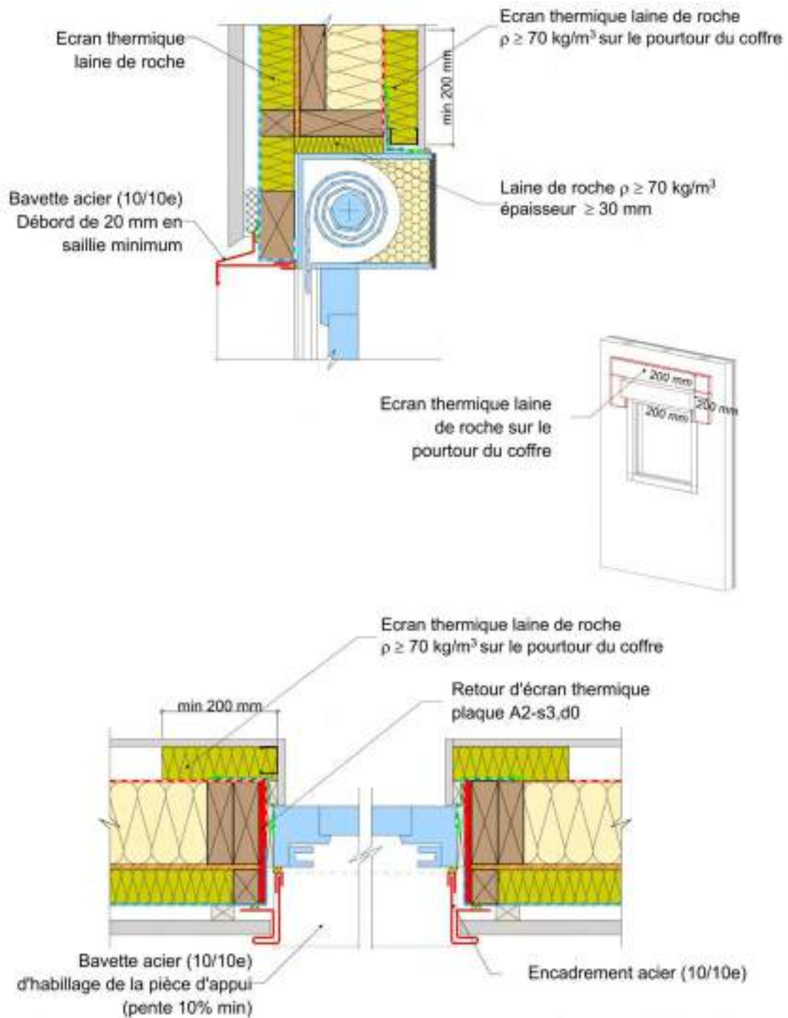
Figure 11: Traitement des baies - menuiseries avec un écran laine de roche + encadrement acier et mise en œuvre d'un coffre de volet roulant.
