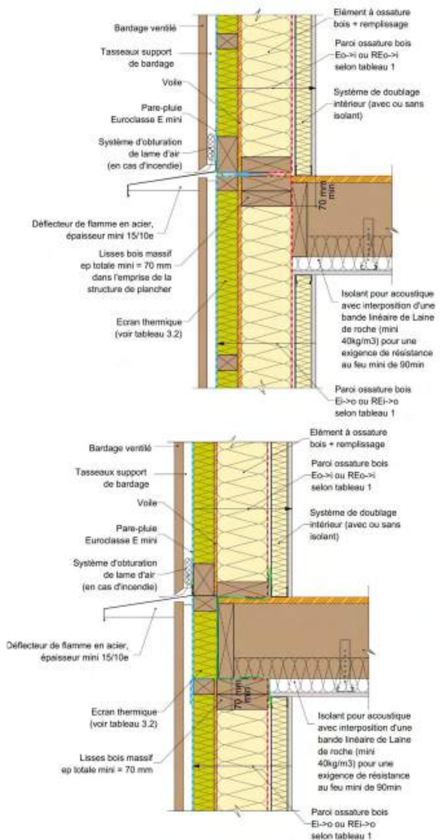
Figure 30 : Façade/mur ossature bois et plancher en ossature bois.
