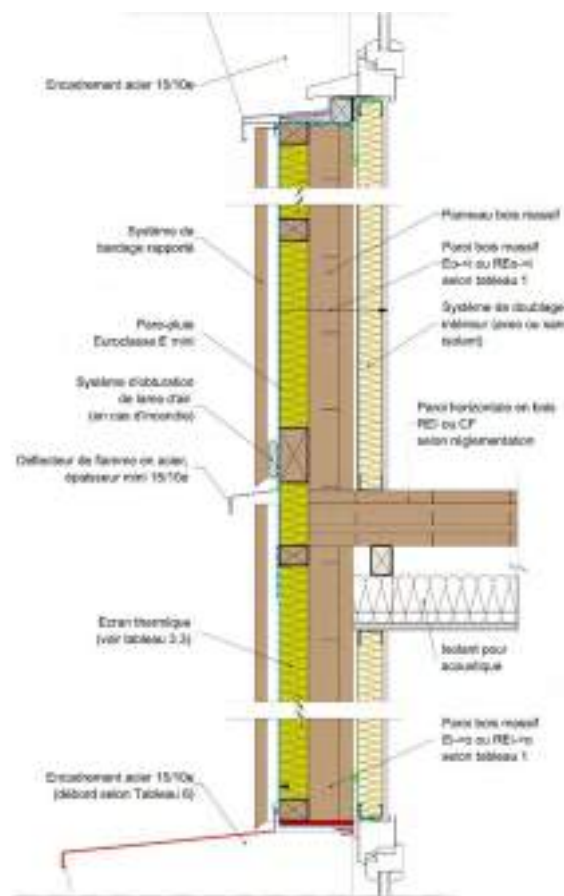
Figure 36 : Façade/mur en ossature bois et plancher en panneaux bois massif.
