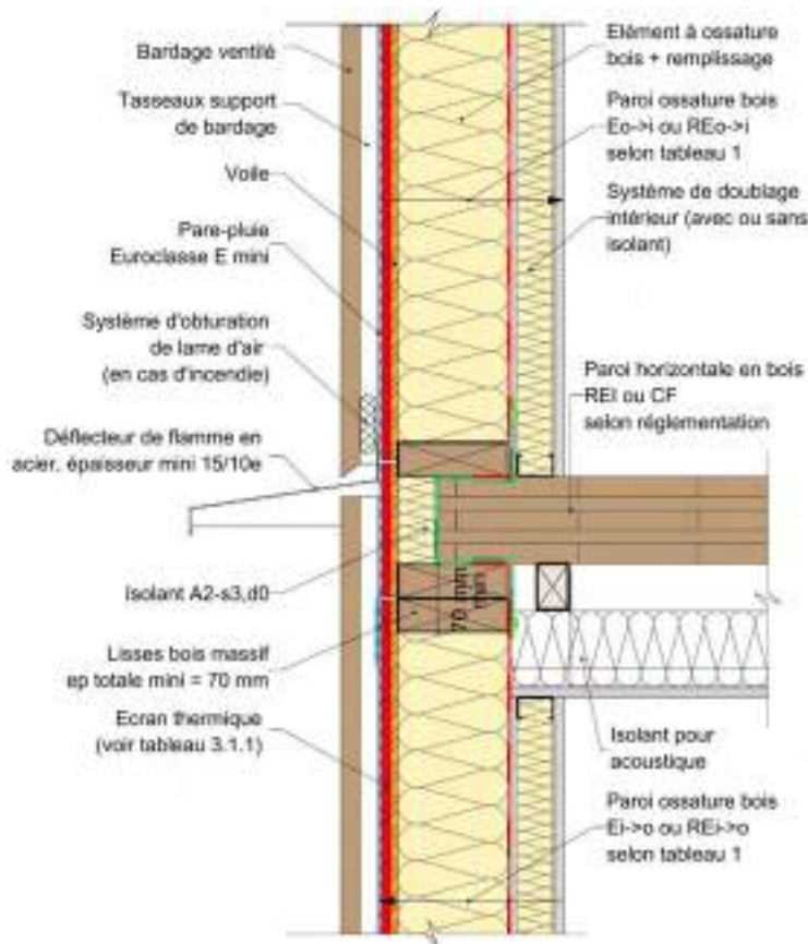
Figure 25 : Façade/mur en ossature bois et plancher en panneau bois massif.
