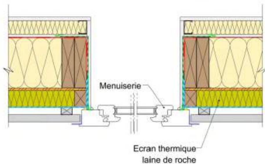
Figure 9: Traitement des baies - menuiseries en applique extérieure avec un écran laine de roche.
