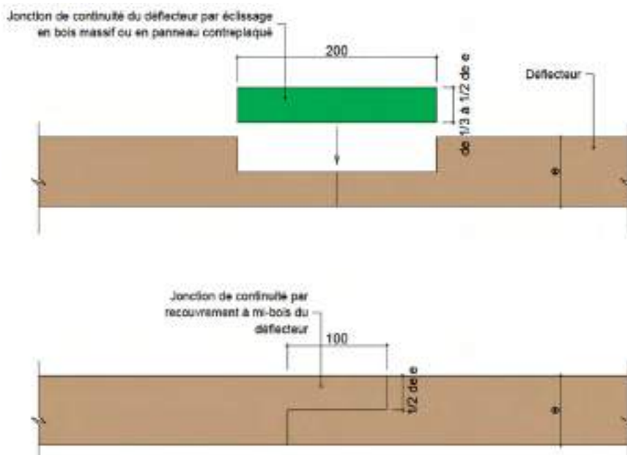
Figure 17 : Continuité du déflecteur bois
