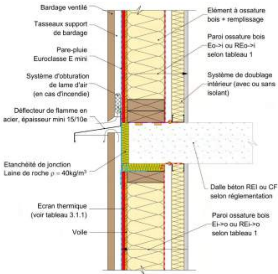
Figure 22 : Façade en ossature bois sur plancher béton.
