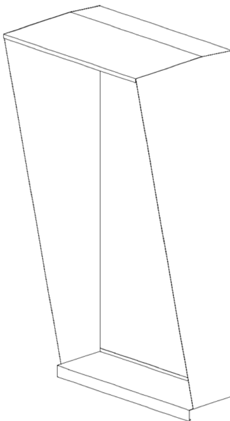
Figure 21 : Habillage des embrasures en acier, en saillie
