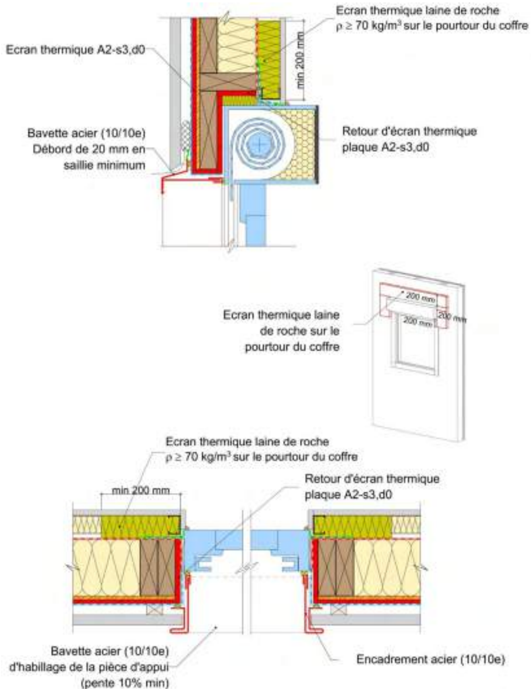
Figure 10: Traitement des baies - menuiseries avec un matériau A2-s3, d0 + encadrement acier et mise en œuvre d'un coffre de volet roulant.
