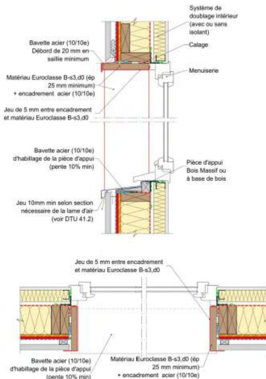
Figure 5: Traitement des baies - menuiseries en applique intérieure avec un matériau B-s3, d0 + encadrement acier.
