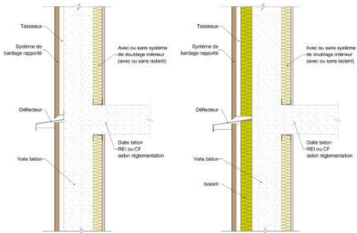
Figure 43 : Bardage ventilé avec revêtement extérieur à base de bois sur support en maçonnerie.
