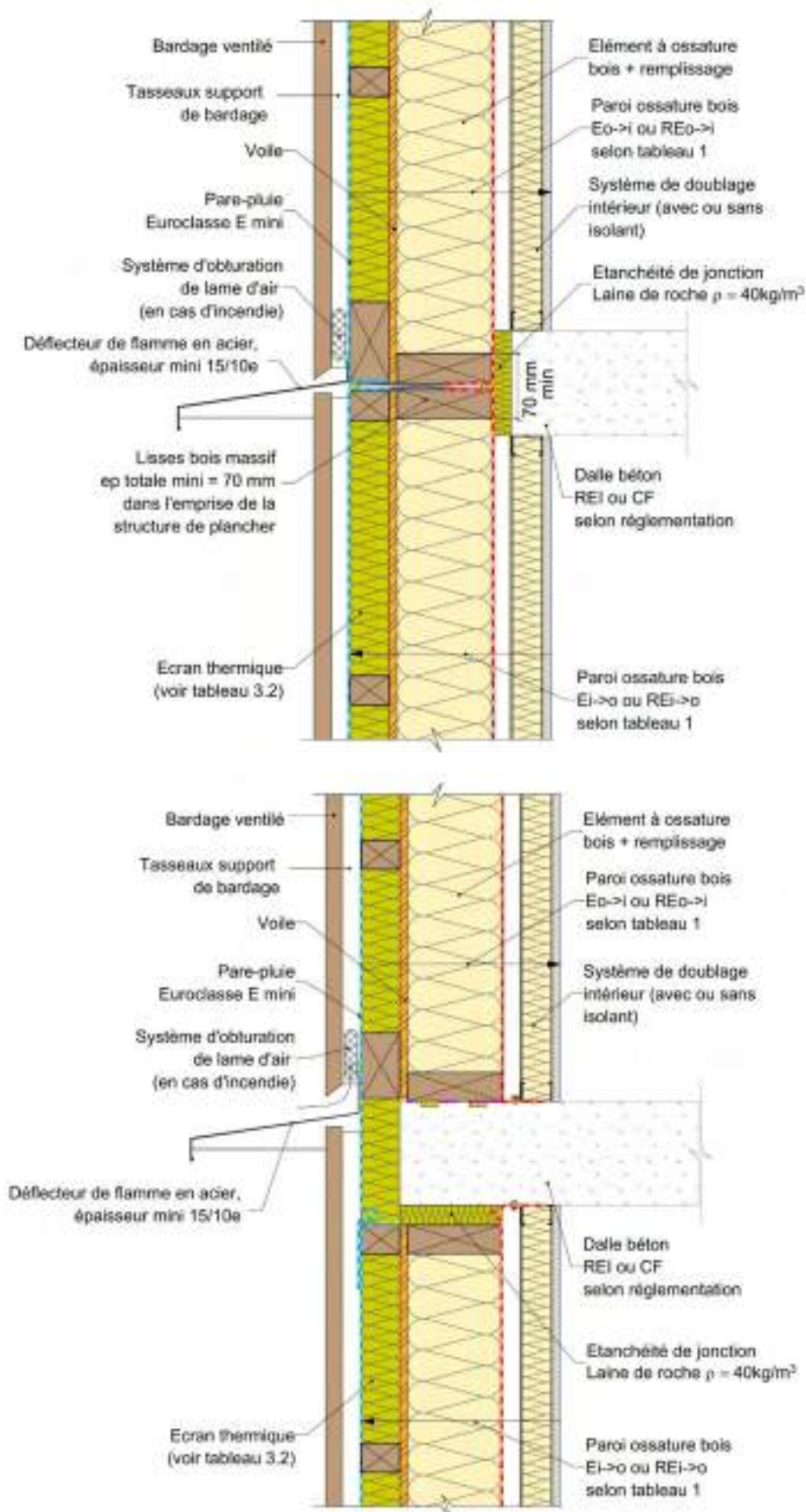
Figure 29 : Façade/mur ossature bois et plancher béton.
