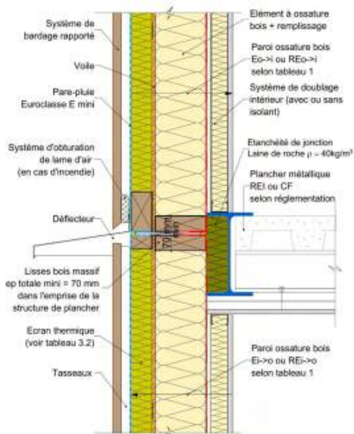
Figure 33 : Façade/mur ossature bois et plancher métallique.
