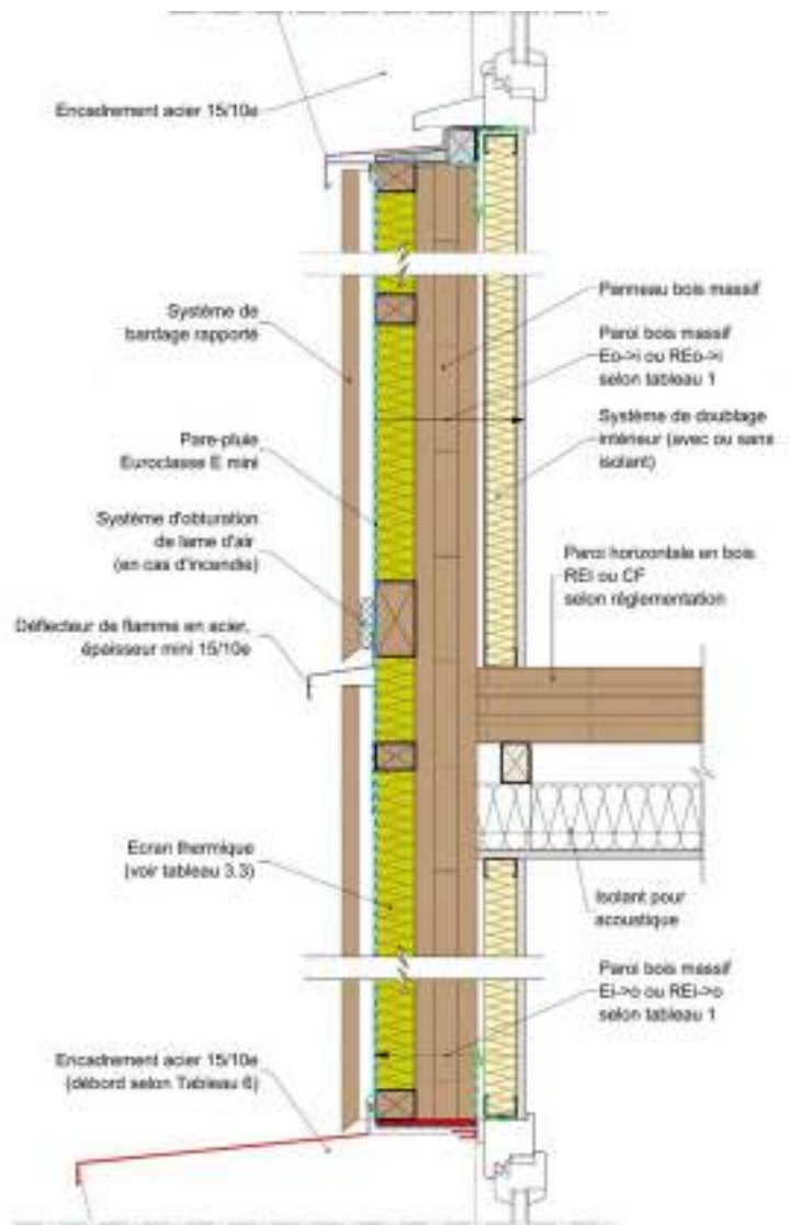
Figure 37 : Façade/mur en panneaux bois massif et plancher en panneaux bois massif.
