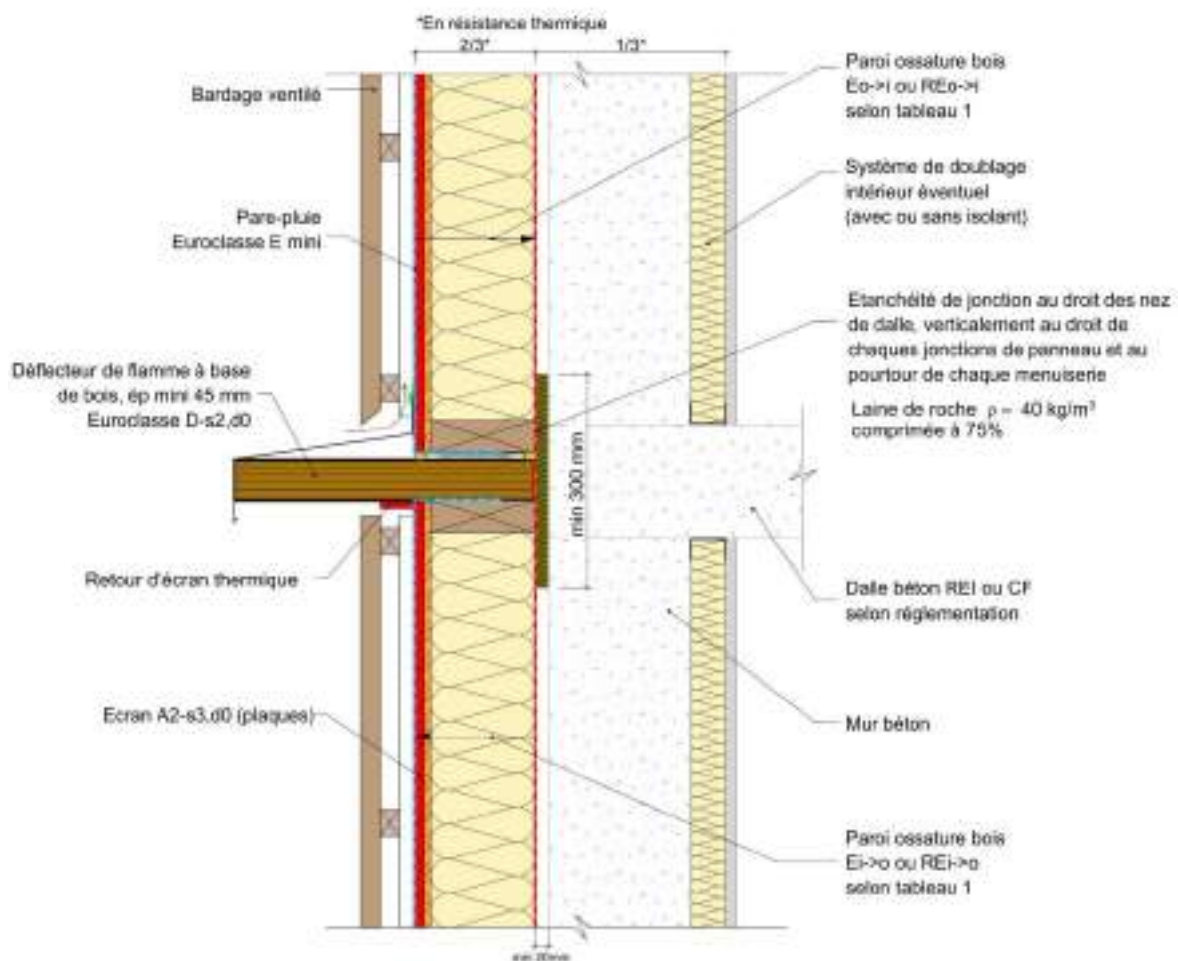
Figure 44 : Système d'isolation thermique par l'extérieur avec revêtement extérieur à base de bois sur support en maçonnerie.
