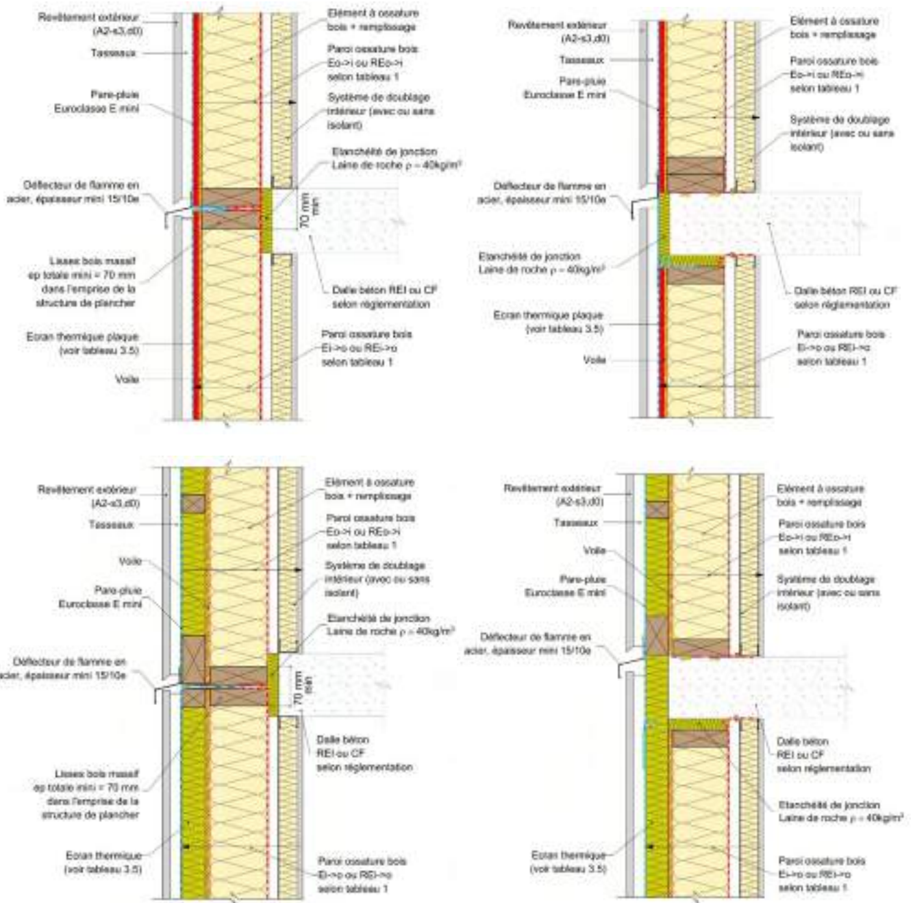
Figure 38 : Façade/mur en ossature bois et plancher en béton.
