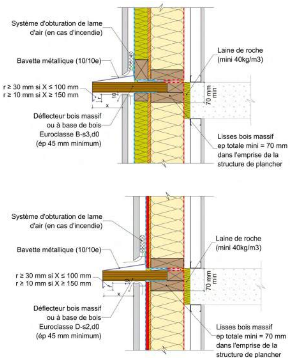
Figure 16: Déflecteur en bois massif ou à base de bois dans le cas où l'écran thermique est réalisé en laine de roche entre ossature (figure du dessus) ou en plaque rigide A2-s3, d0 (figure du dessous).
