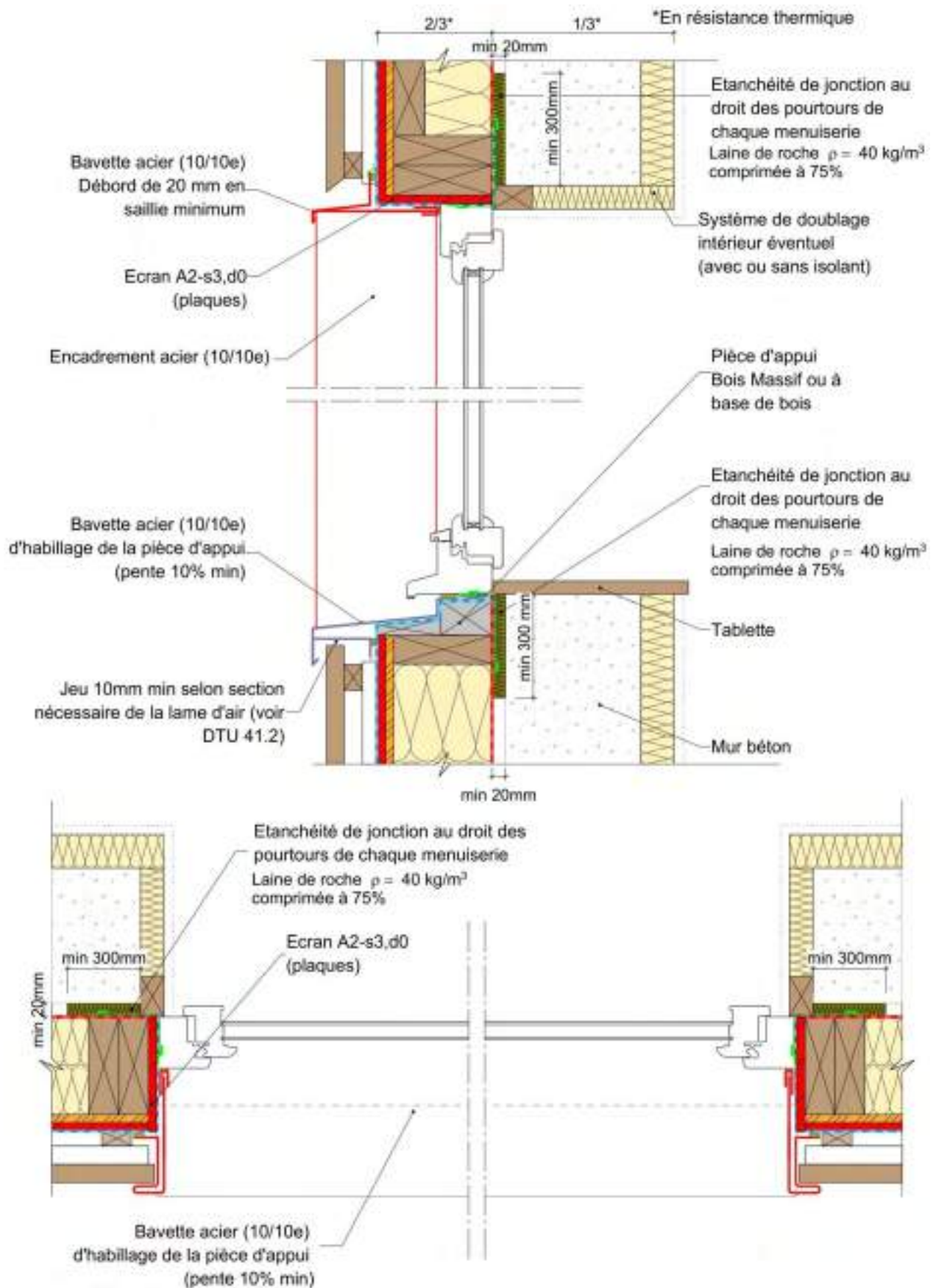
Figure 45 : Système d'isolation thermique par l'extérieur avec revêtement extérieur à base de bois sur support en maçonnerie – détails de baies
