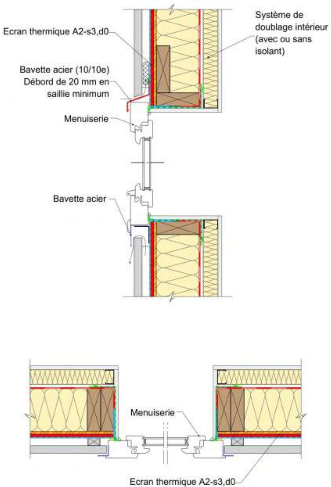
Figure 8: Traitement des baies - menuiseries en applique extérieure avec un matériau A2-s3, d0.
