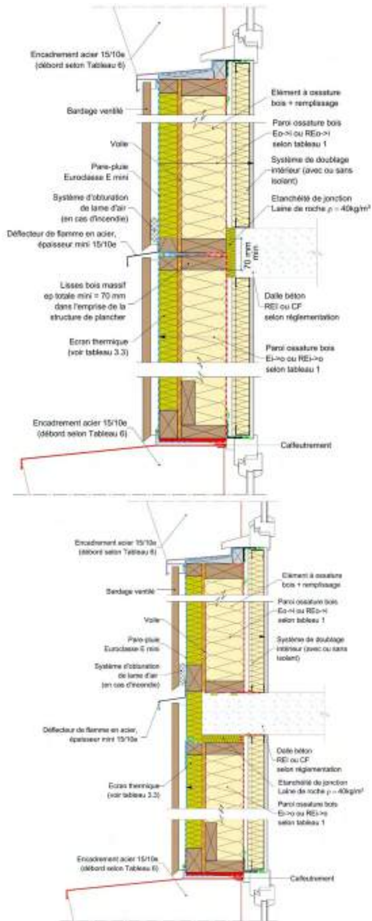
Figure 34 : Façade/mur ossature bois et plancher en béton.
