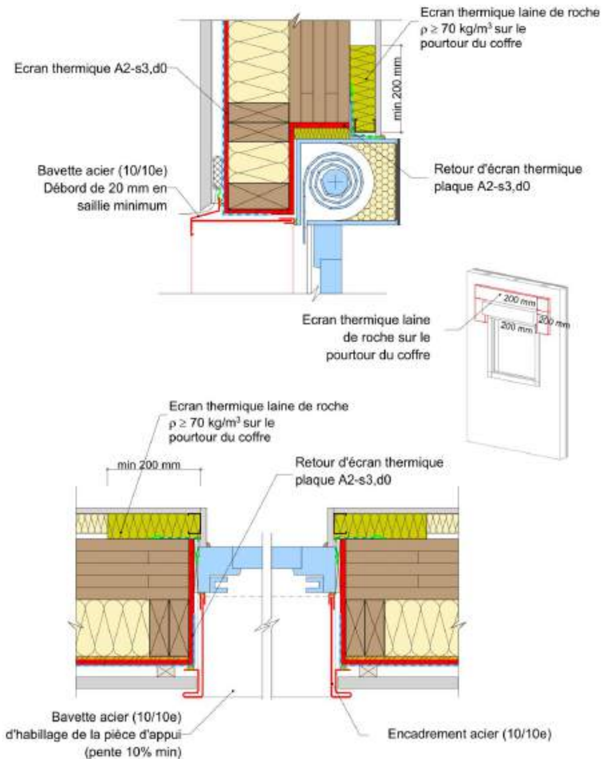
Figure 12: Traitement des baies - menuiseries sur panneaux bois massif contrecollés et contrecloués avec un écran laine de roche + encadrement acier et mise en œuvre d'un coffre de volet roulant.
