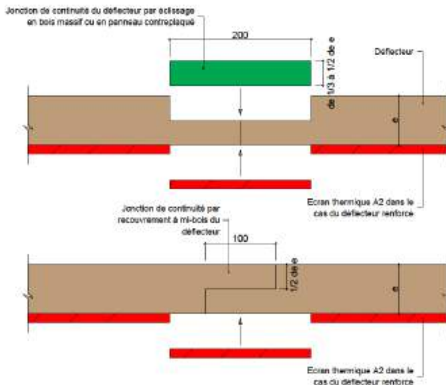
Figure 19 : Jonction du déflecteur bois renforcé
