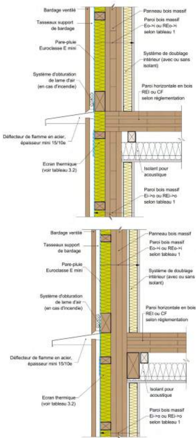
Figure 31 : Façade/mur en panneaux bois massif et plancher en panneau bois massif.
