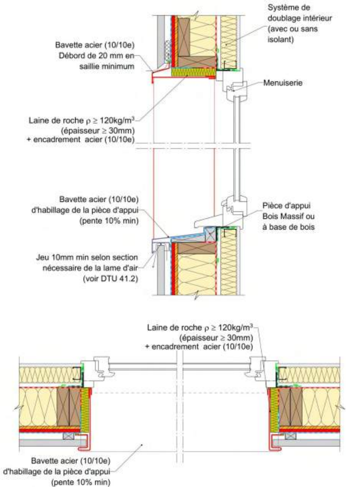
Figure 7: Traitement des baies - menuiseries en applique intérieure avec un écran laine de roche + encadrement acier.
