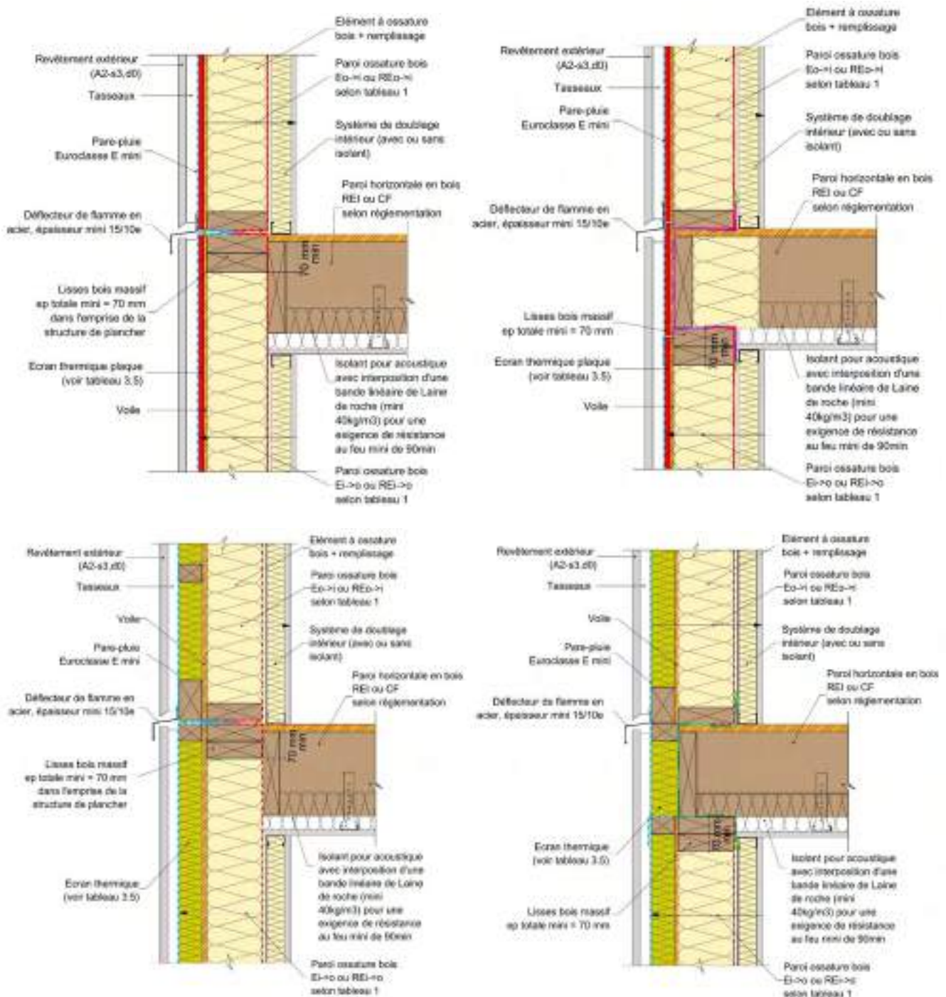
Figure 39 : Façade/mur en ossature bois et plancher en ossature bois.
