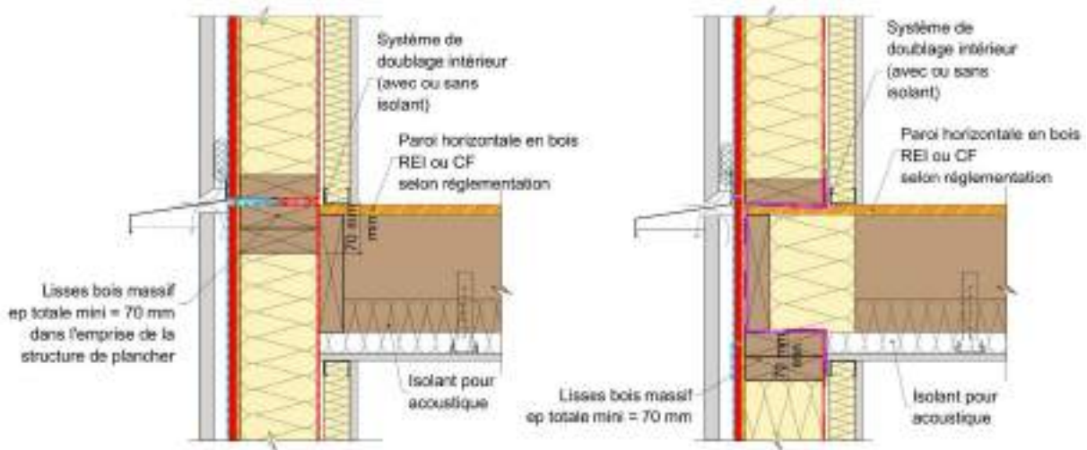
Figure 3: Traitement de l'étanchéité au nez d'un plancher bois avec doublage intérieur assurant l'intégralité de l'exigence EI_{i \rightarrow o} requise et au moins égale à la performance du plafond (si la durée de résistance au feu de la structure est inférieure ou égale à 60 minutes).
