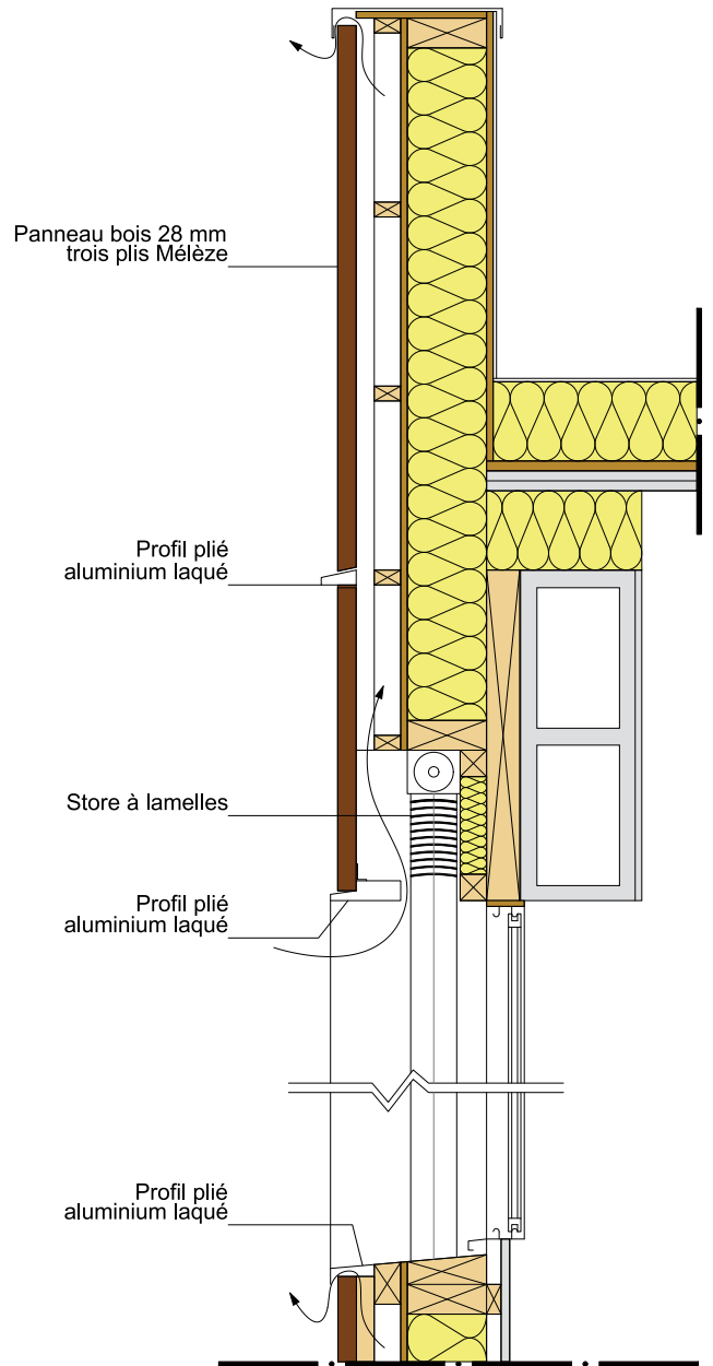
Coupe verticale
