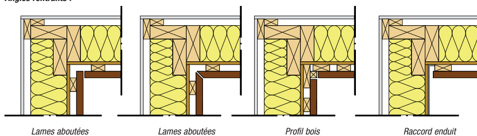
Lames aboutées
