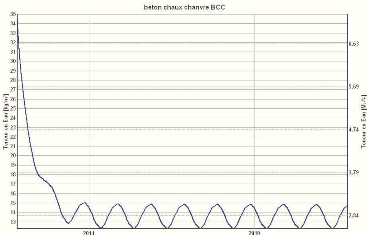
Etude WUFI : Teneur en eau du béton de chanvre
