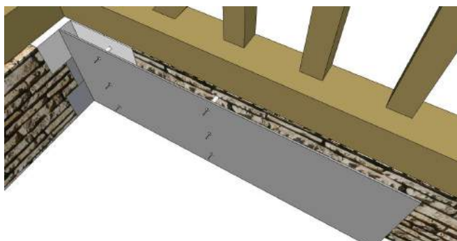
Pose de banche au niveau du soubassement du pan de bois
