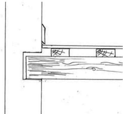
Coupe About de poutre - Source : maison paysanne
