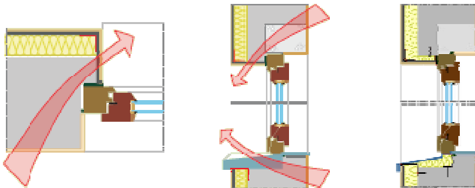
Ponts thermiques au niveau de l'encadrement.
