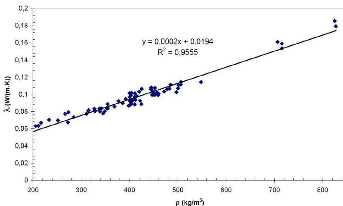
La conductivité thermique du béton de chanvre sec en fonction de la masse volumique (Cérézo, 2008).
