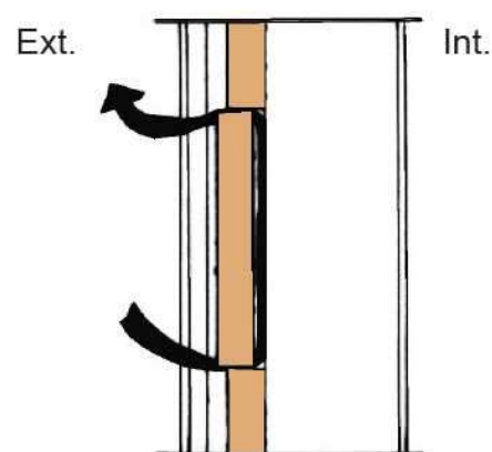
Étanchéité à l'air pour ITE ; Source ADEME
