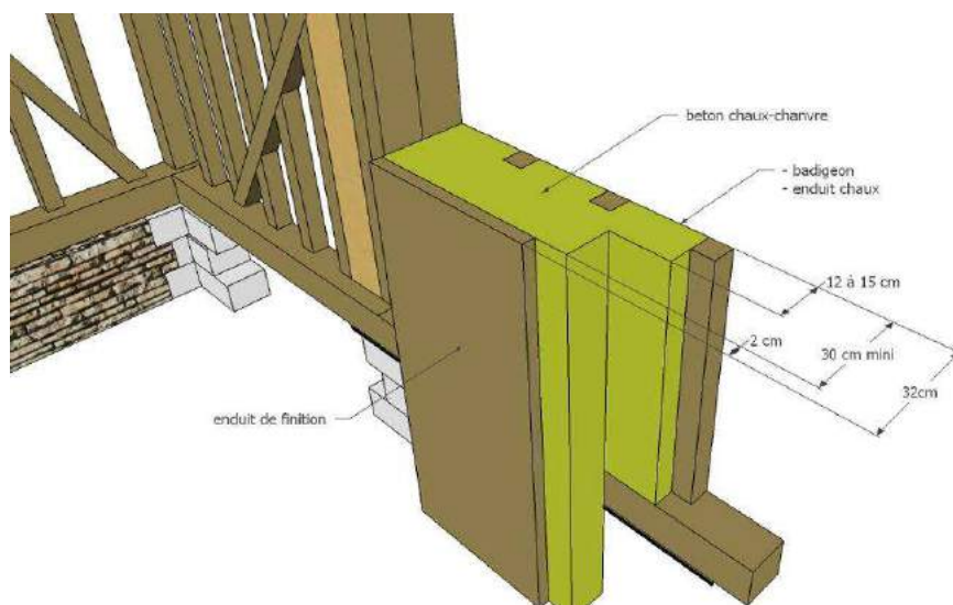
Isolation répartie d'un pan de bois
