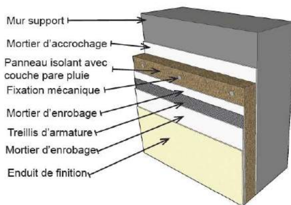
Isolation par l'extérieur. Source ADEME
