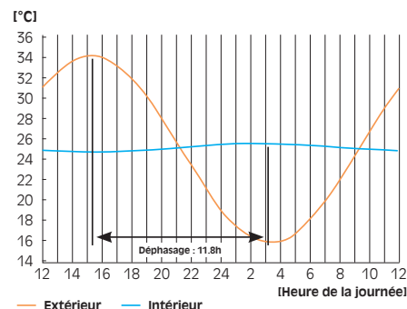
La courbe rouge présente l'évolution de la température d'une journée d'été. La courbe bleue présente le déphasage de l'onde de chaleur et la réduction de son amplitude.
