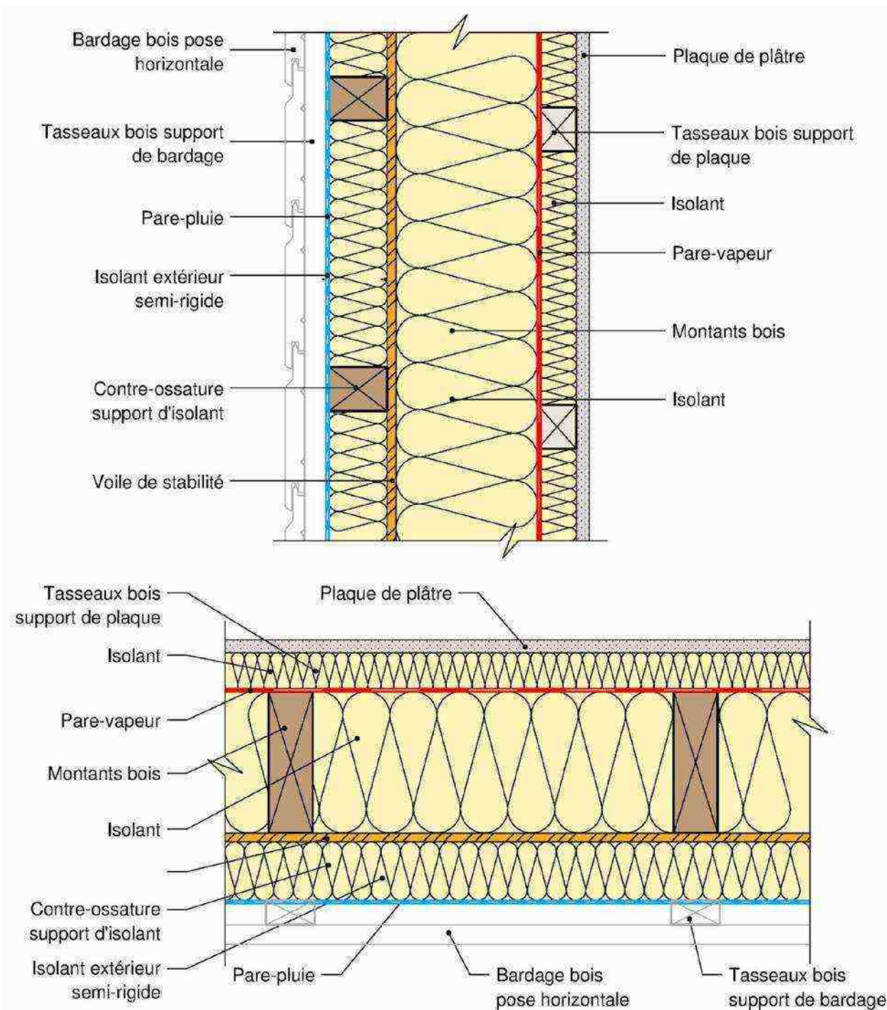
▲ Figure 23 : Coupe verticale (haut) et coupe horizontale (bas) d'une façade ossature bois avec isolation en âme et complément isolant intérieur et extérieur
