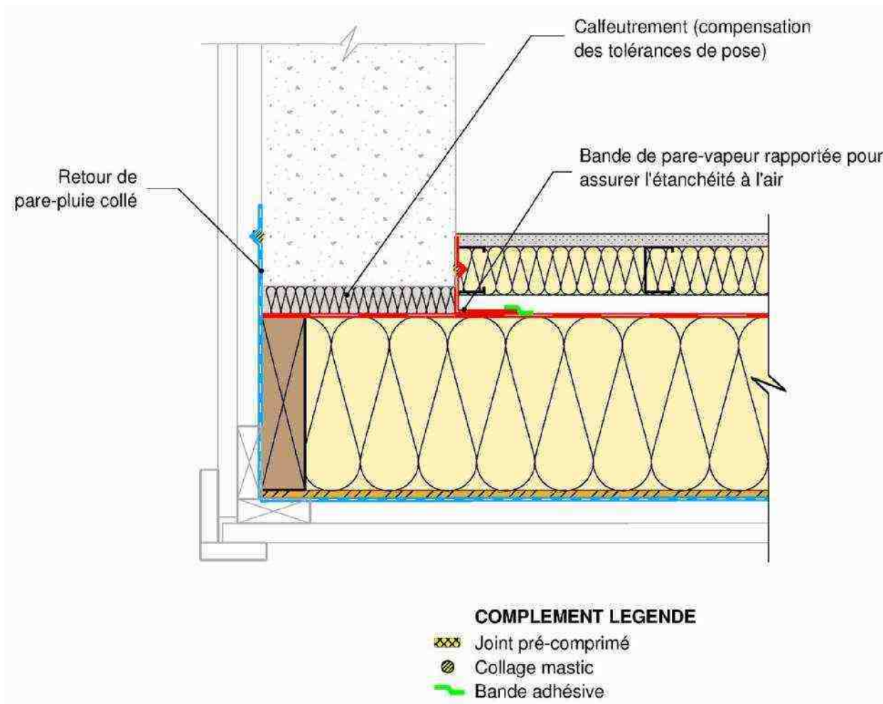
▲ Figure 19 : Assemblage en angle avec mur pignon béton – Coupe horizontale sur pignon
