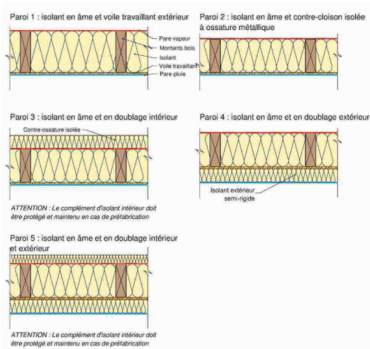
▲ Figure 42 : Eléments inclus dans un allotissement de type SE pour chaque type de paroi courante
