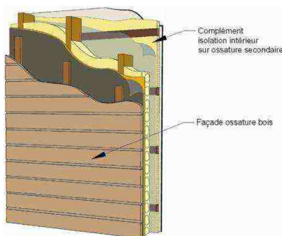
▲ Figure 3 : Complément d'isolation intérieur rapporté sur ossature principale
