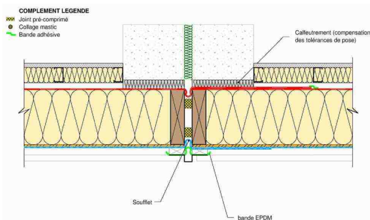
▲ Figure 21 : Gestion des joints de dilatation – Coupe horizontale
