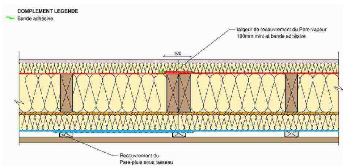
▲ Figure 8 : Coupe horizontale – Recouvrement vertical du pare-pluie souple
