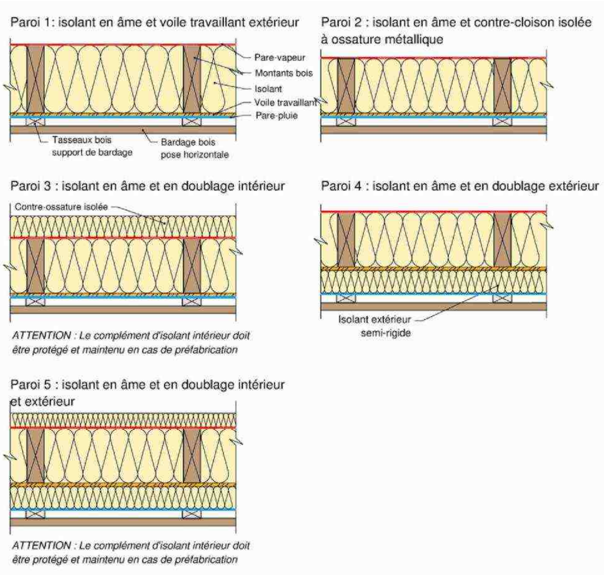
▲ Figure 43 : Éléments inclus dans un allotissement de type SER pour chaque type de paroi courante
