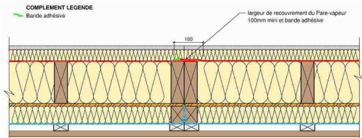
▲ Figure 9 : Coupe horizontale – Recouvrement vertical du pare-pluie souple dans le cas de panneaux préfabriqués
