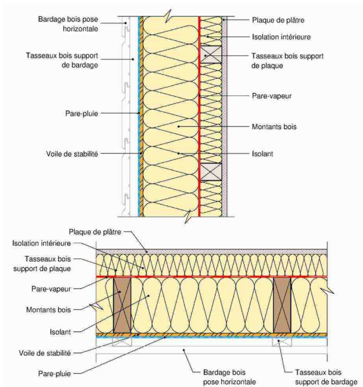
▲ Figure 11 : Coupe verticale (haut) et coupe horizontale (bas) d'une façade ossature bois avec isolation en âme et complément isolant par l'intérieur
