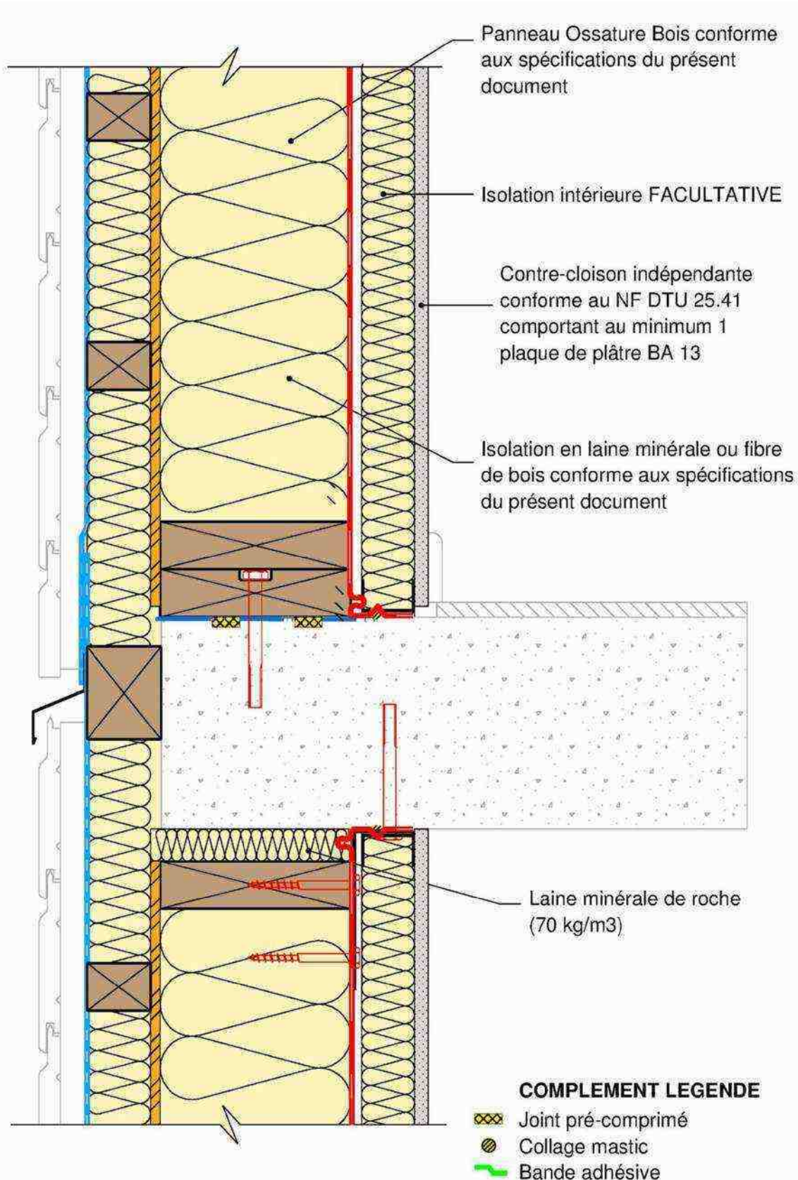
▲ Figure 34 : Coupe verticale d'une liaison plancher / façade semi-filante
