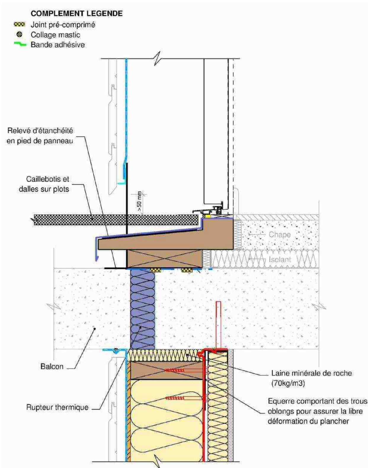
▲ Figure 30 : Porte-fenêtre sur balcon – Coupe verticale
