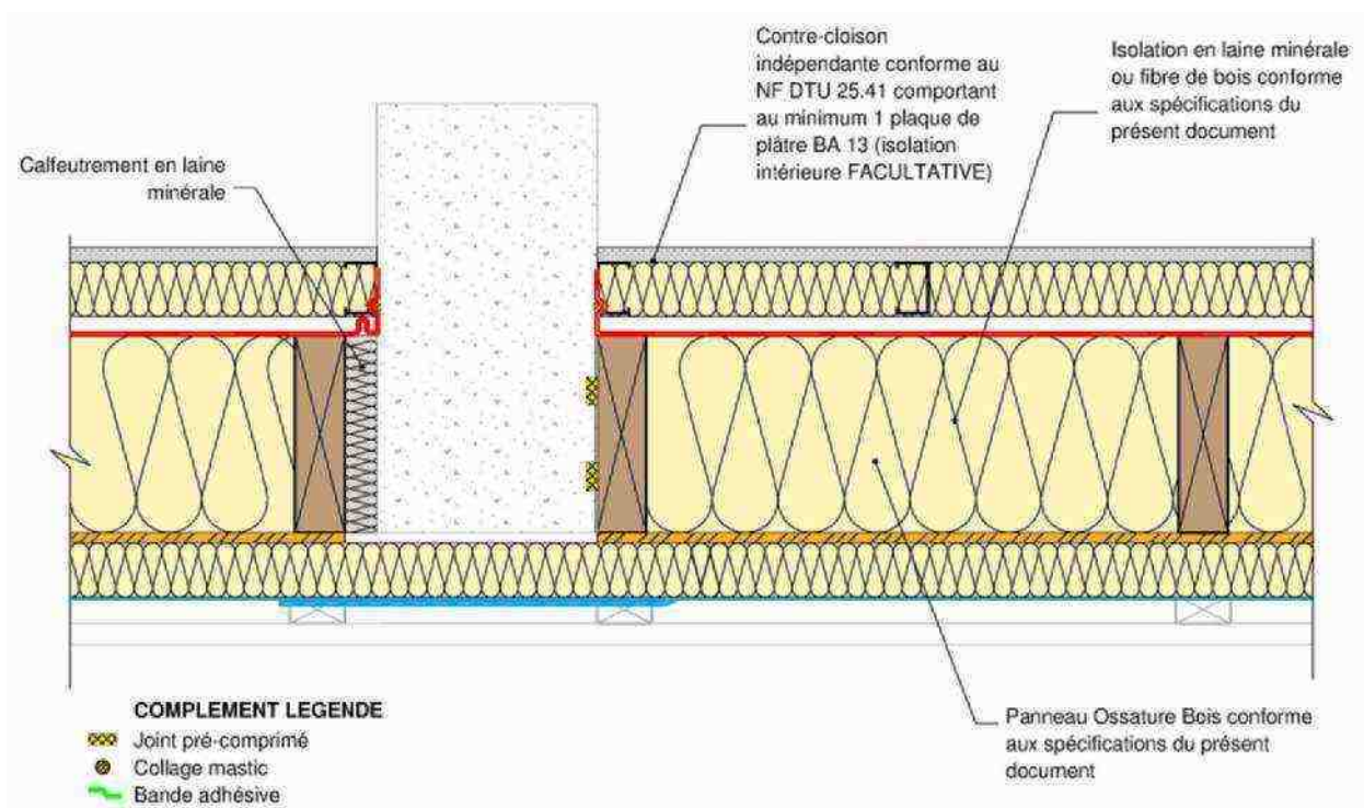
▲ Figure 35 : Coupe horizontale d'une liaison refend / façade semi-filante
