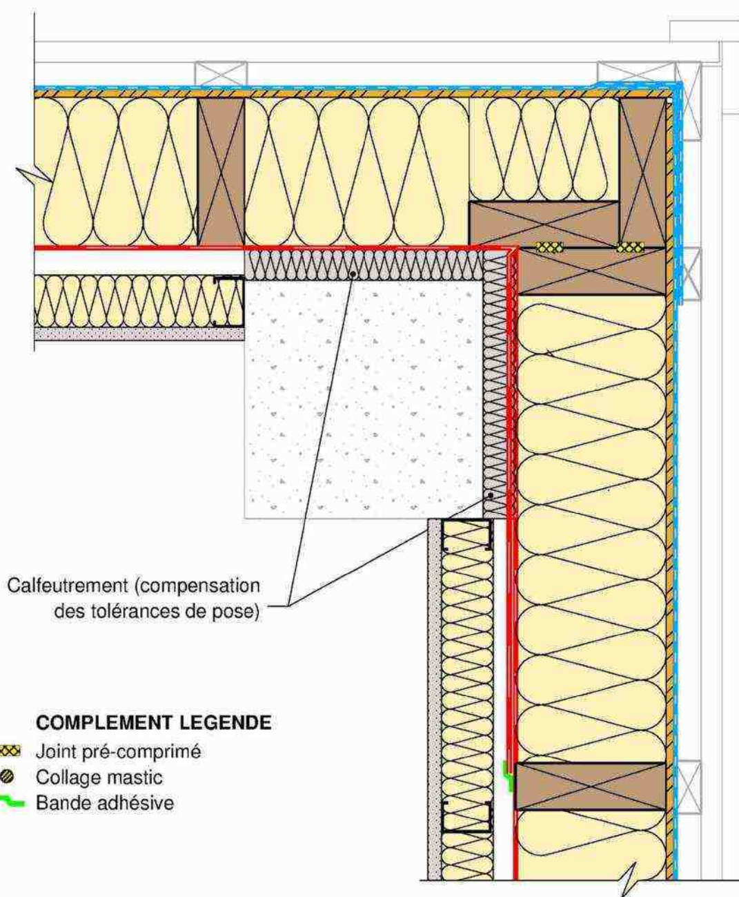
▲ Figure 17 : Assemblage en angle sortant – Coupe horizontale sur poteau
