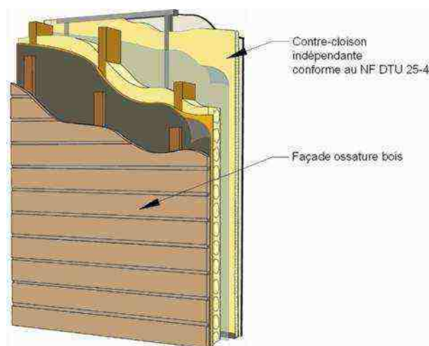
▲ Figure 4 : Contre-cloison rapportée indépendamment de l'ossature principale
