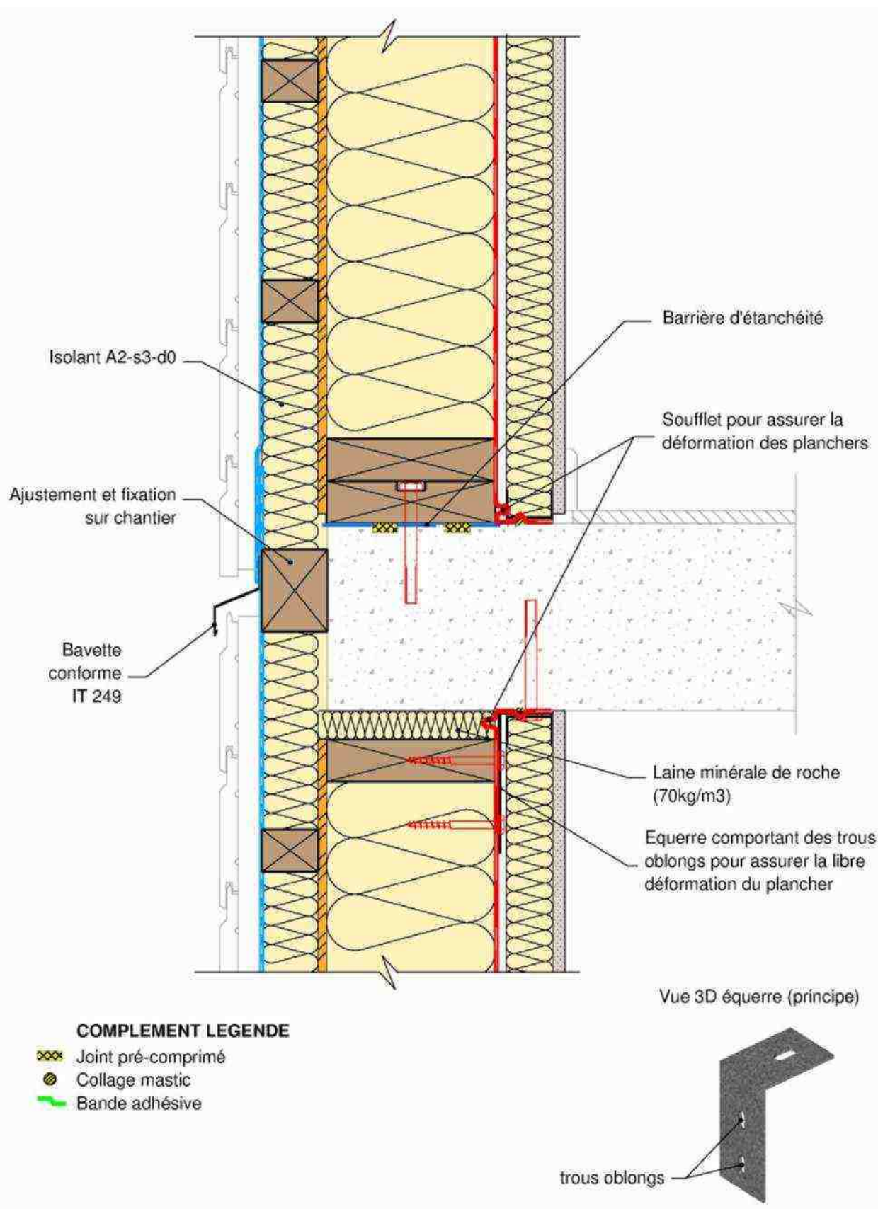
▲ Figure 24 : Fixation en pied et en tête des façades semi-filantes – Coupe verticale
