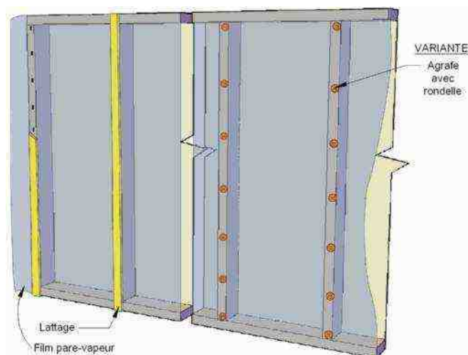
▲ Figure 6 : Fixation définitive du pare-vapeur dans le cas d'une contre-cloison indépendante
