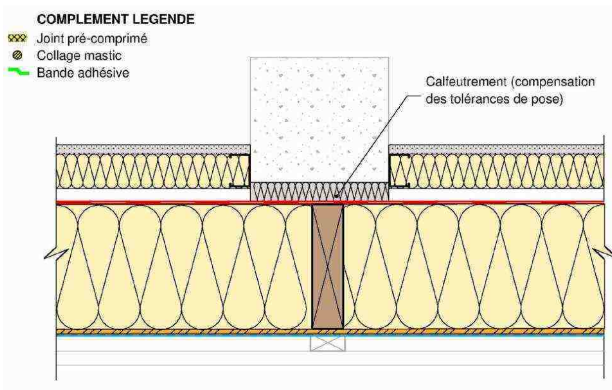
▲ Figure 16 : Liaison avec les porteurs verticaux / Configuration de façade filante – Coupe horizontale sur poteau
