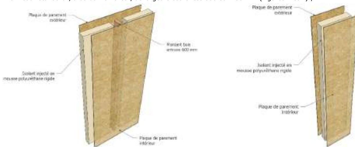
Figure 1 – Vue éclatée d'un "Panneau Standard LogiPanel®" 1200 mm Figure 2 – Vue éclatée d'un "Panneau Standard LogiPanel®" 600 mm
