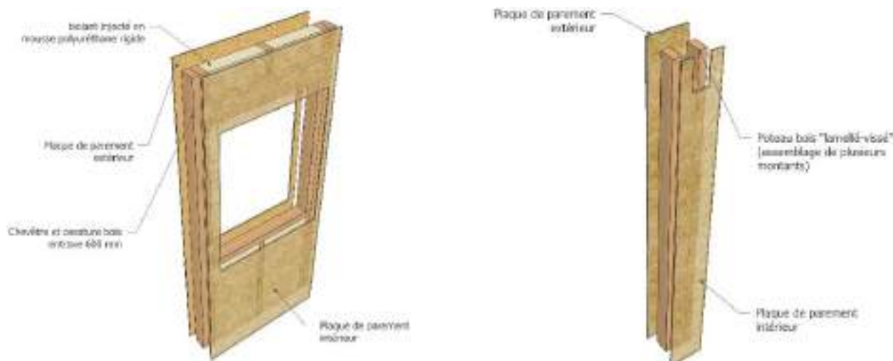
Figure 3 – Vue éclatée d'un "Panneau Menuisé LogiPanel®"
