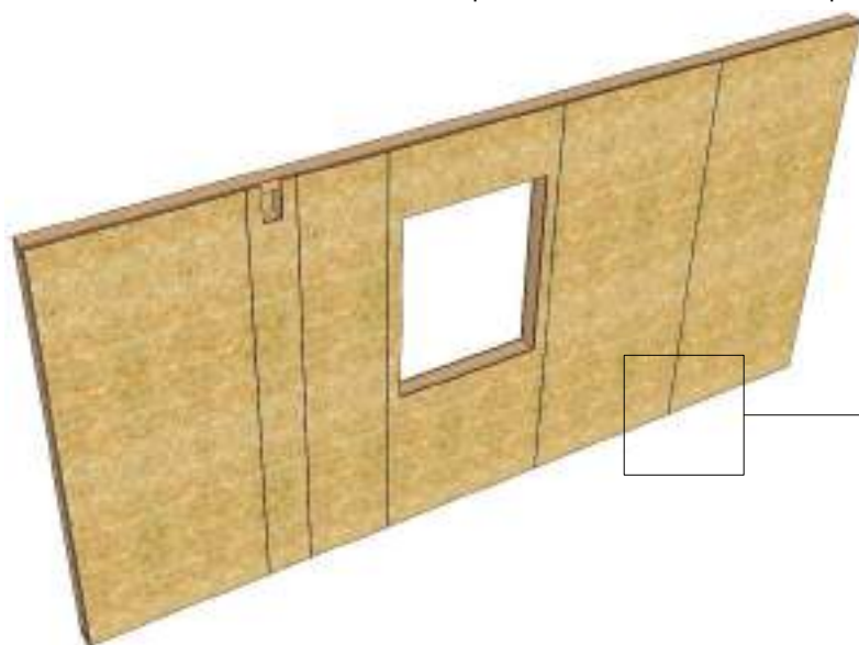
Figure 6 - Couturage d'un panneau de mur LogiWall®
