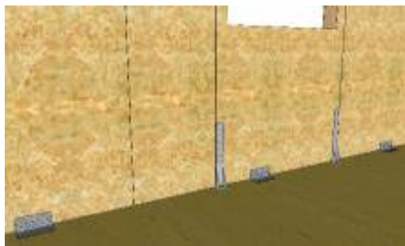
Figure 20 – Mise en œuvre des équerres anti-soulèvement en pied de panneau de mur et en sous face de plancher
