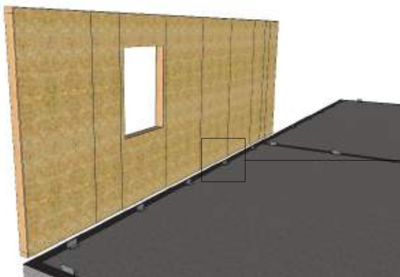
Figure 11 – Approche du panneau de mur LogiWall® / Guidage et mise en position des panneaux de mur en appui contre les équerres de reprise du glissement
