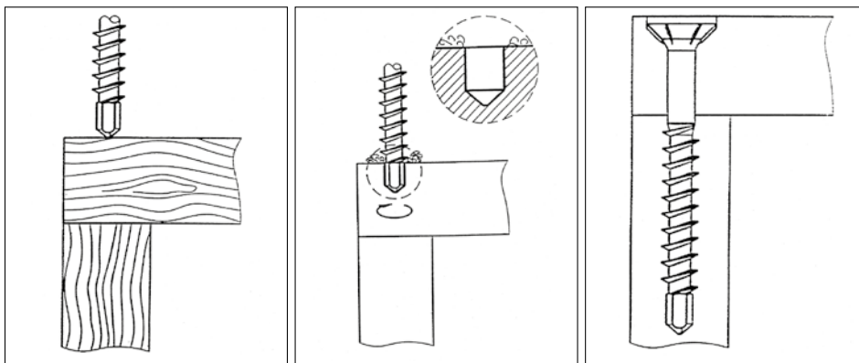
Sans pré-perçage grâce à la pointe auto-perceuse.
